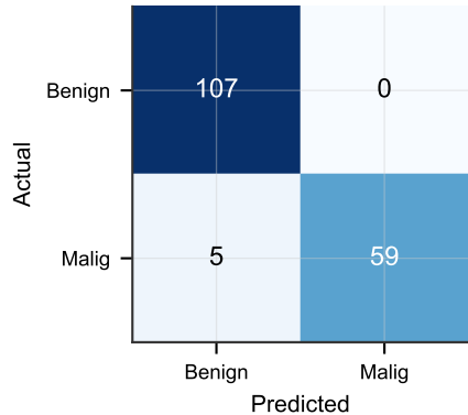
SVM
