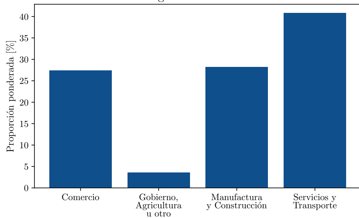
Asignación dura final
