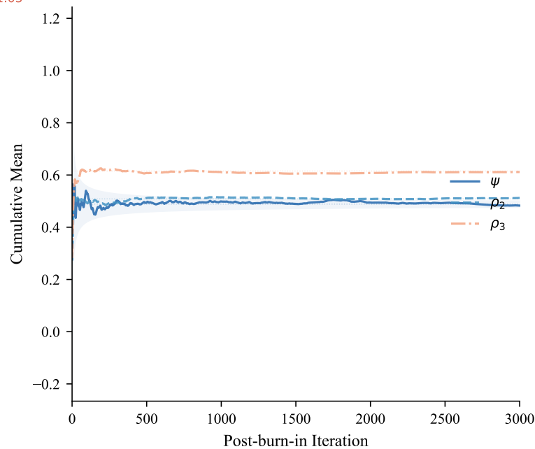
(d) Cumulative Posterior Mean Convergence
