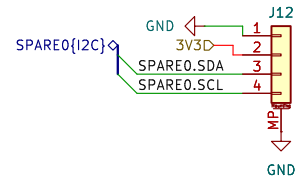
STEMMA QT Connector
