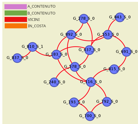
Figura 4.7: Grafo cluster principale dei VICINI
