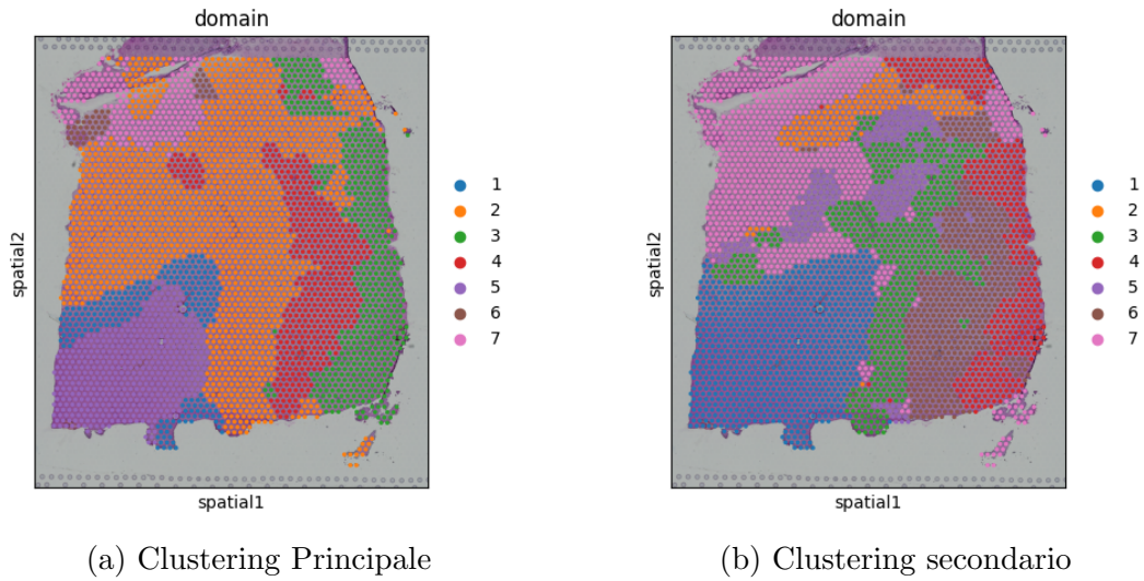
Figura 5.2: Rappresentazione Mclust su AnnData filtrati coi geni in rapporto VICINI
