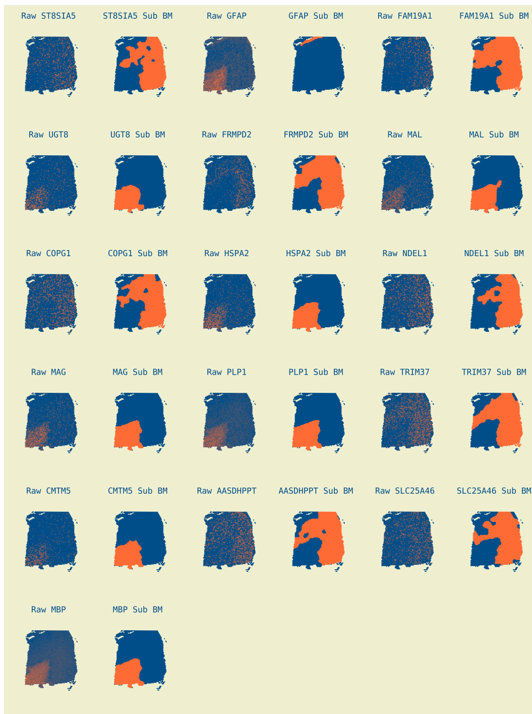
Figura 4.10: Rappresentazione maschere binarie cluster primario
