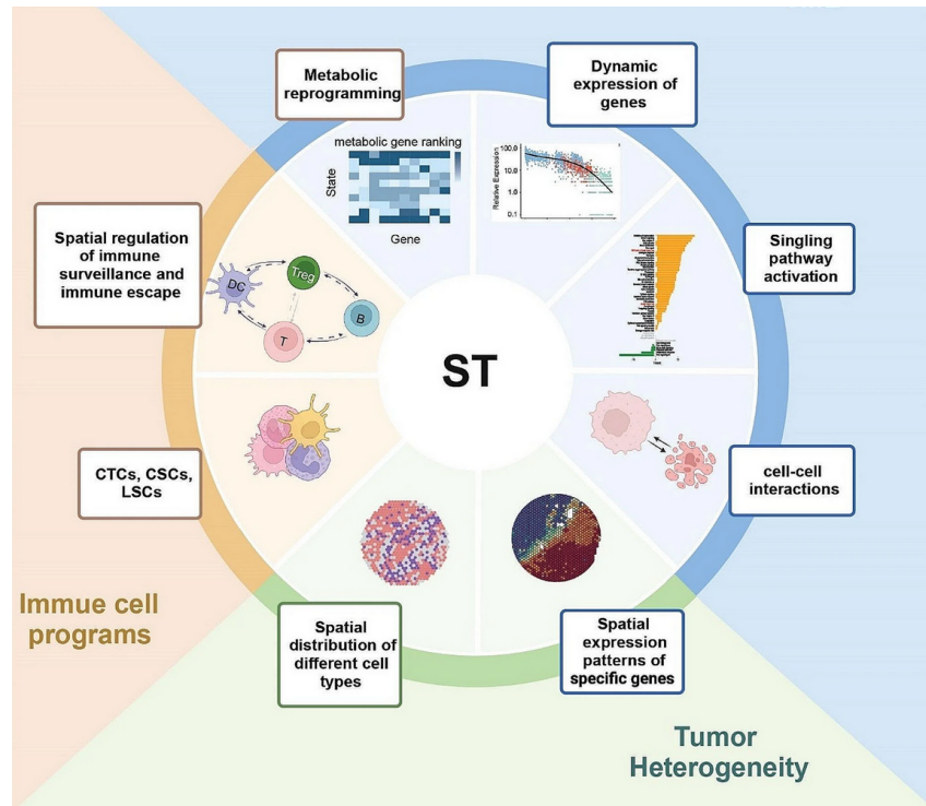
Figura 2.3: Applicazione della trascrittómica spaziale nella ricerca sul cancro
