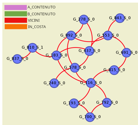
Figura 4.8: Grafo cluster principale dei VICINI
