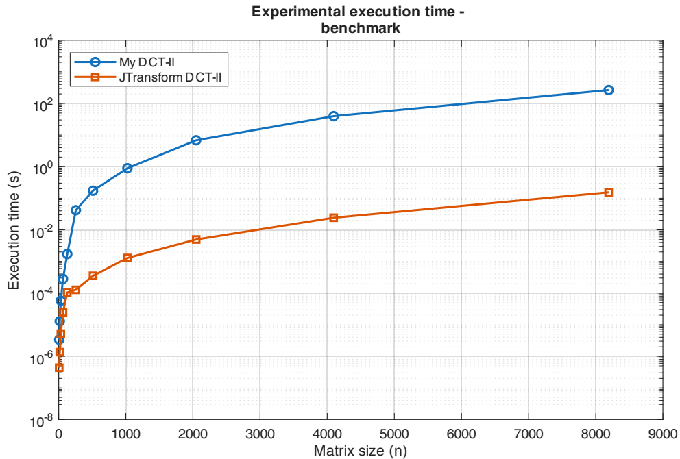
Figura 1.1: Risultati del benchmark tra la nostra implementazione della DCT2 e quella fornita da JTransform
