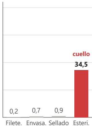
3 réplicas de envasado
