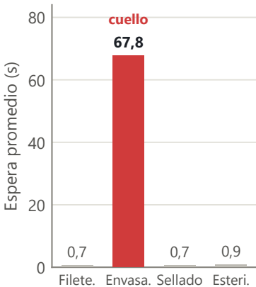
1 réplica de envasado
