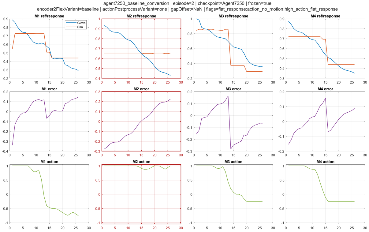
Figure 18: Figura MATLAB forense, baseline, episodio 2 con flags de motor 2.
