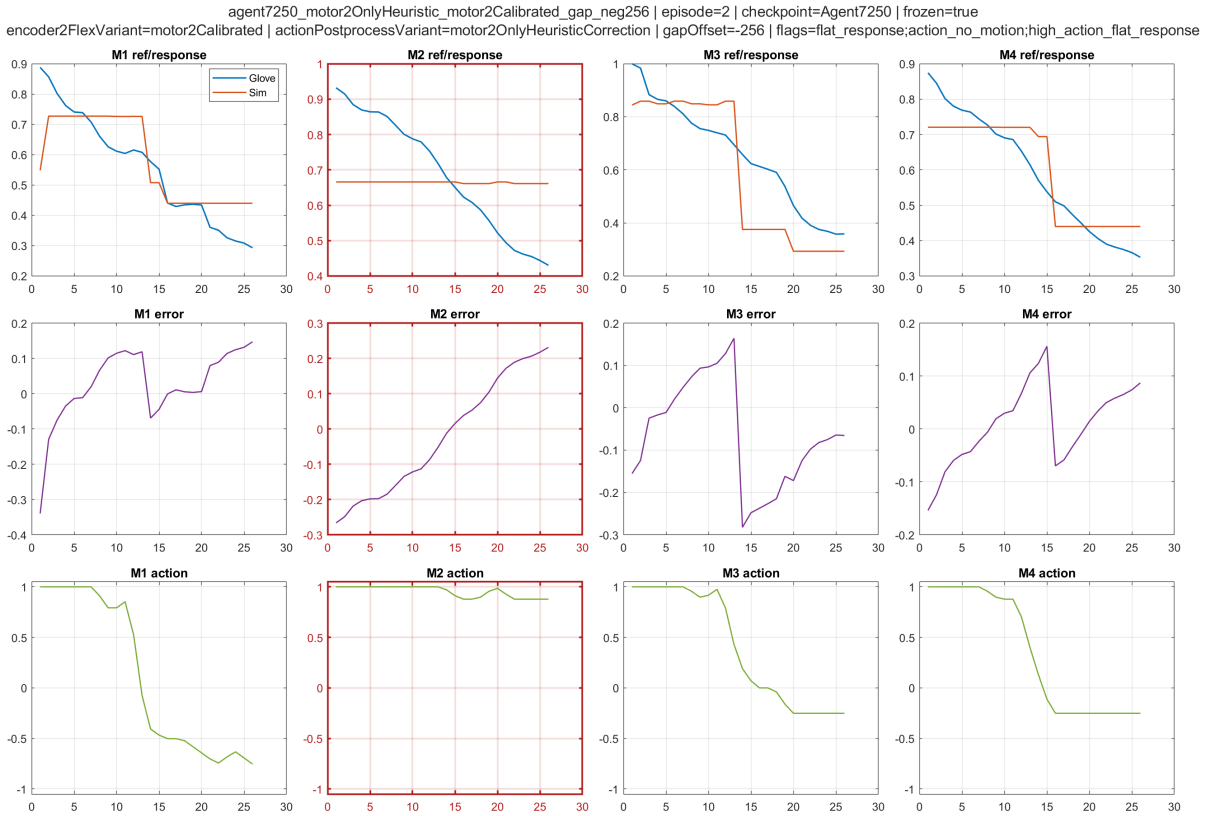
Figure 19: Figura MATLAB forense, heuristica M2-only con conversion calibrada, episodio 2 con flags de motor 2.
