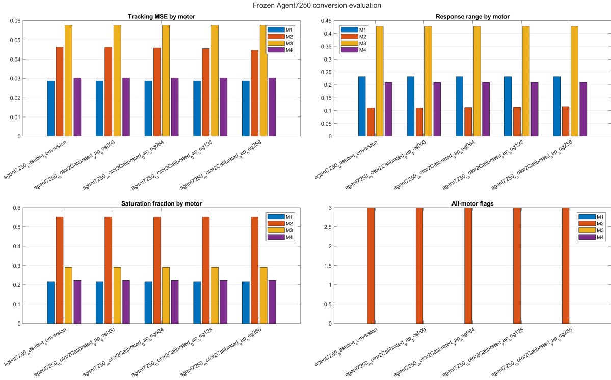
Figure 13: Comparacion MATLAB all-motor con Agent7250 congelado.
