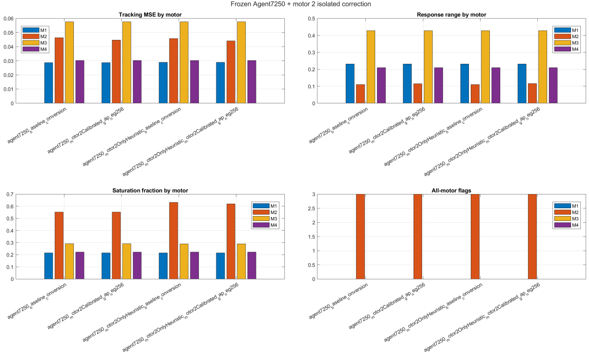
Figure 14: Comparacion MATLAB all-motor con correccion aislada de motor 2.
