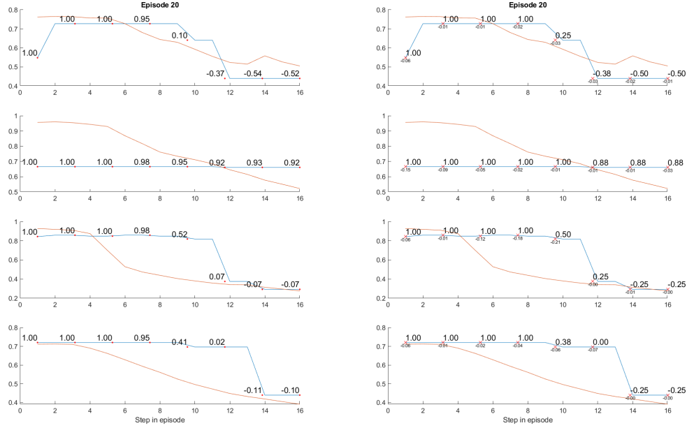
Figure 15: Test visual MATLAB, episodio 20, Agent7250 congelado con correccion aislada de motor 2 y conversion calibrada.
