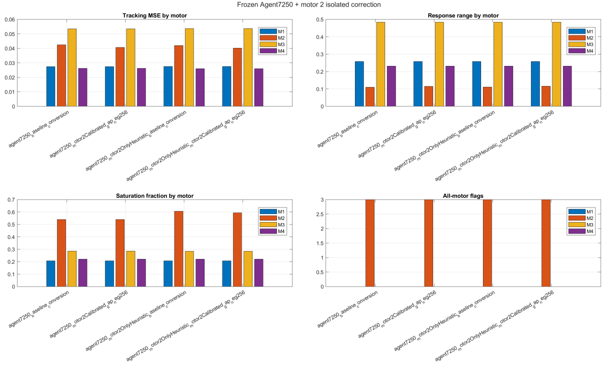
Figure 14: Comparacion MATLAB all-motor con correccion aislada de motor 2, 50 episodios.
