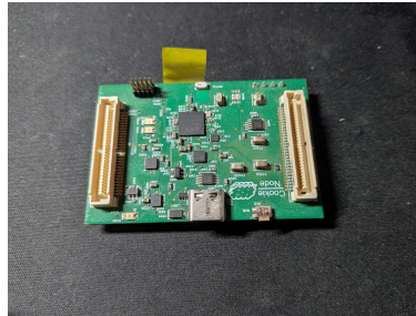
(a) Nodo embebido Cookie.
