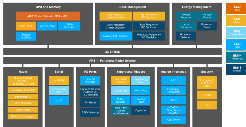
(a) Nodo embebido Cookie.
