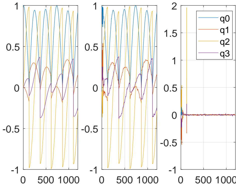
Comparação quatérnion verdadeiro e quatérnion propagado - C
