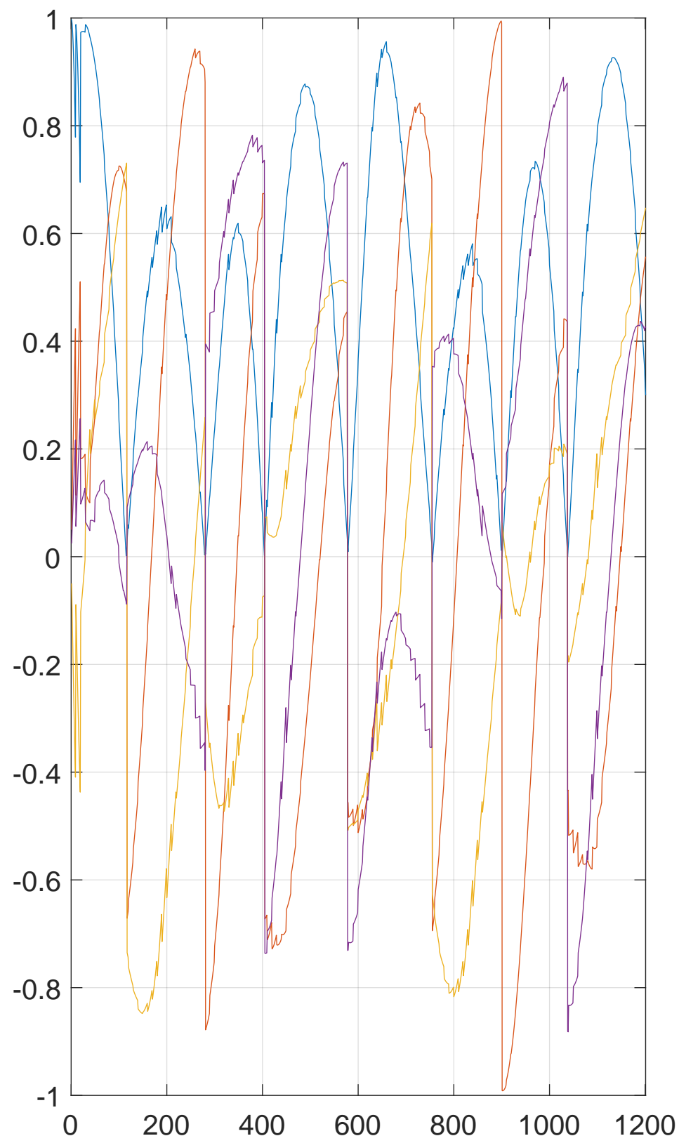
Comparação quatérnio verdadeiro e quatérnio estimado - C
