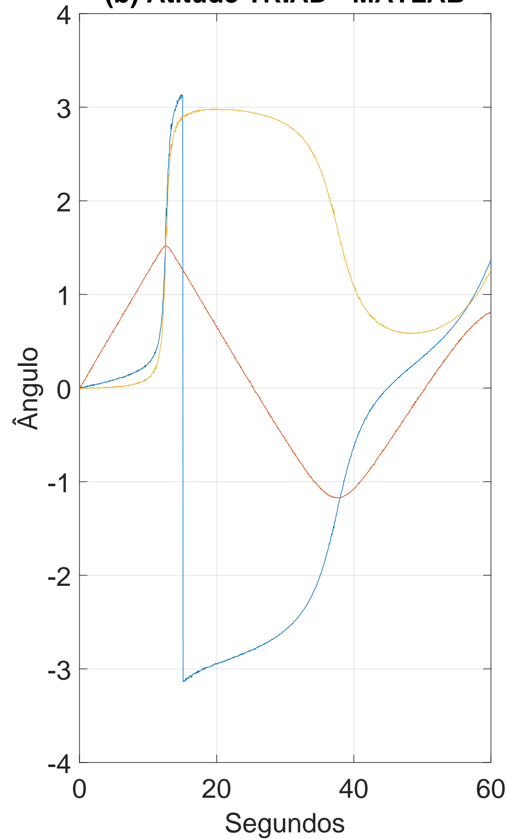
(b) Atitude TRIAD - MATLAB
