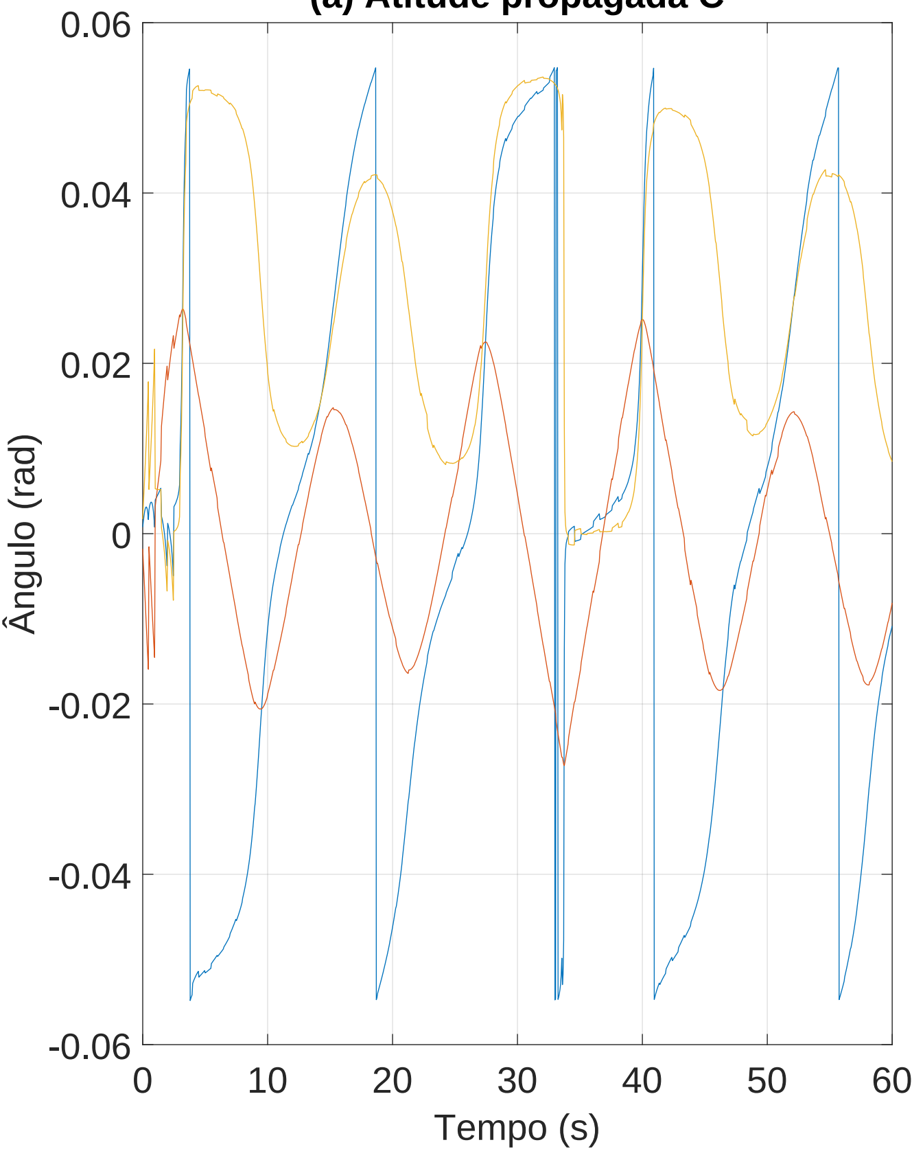
(a) Atitude propagada C
