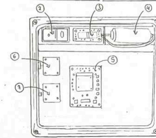
Vista Superior (Componentes)
