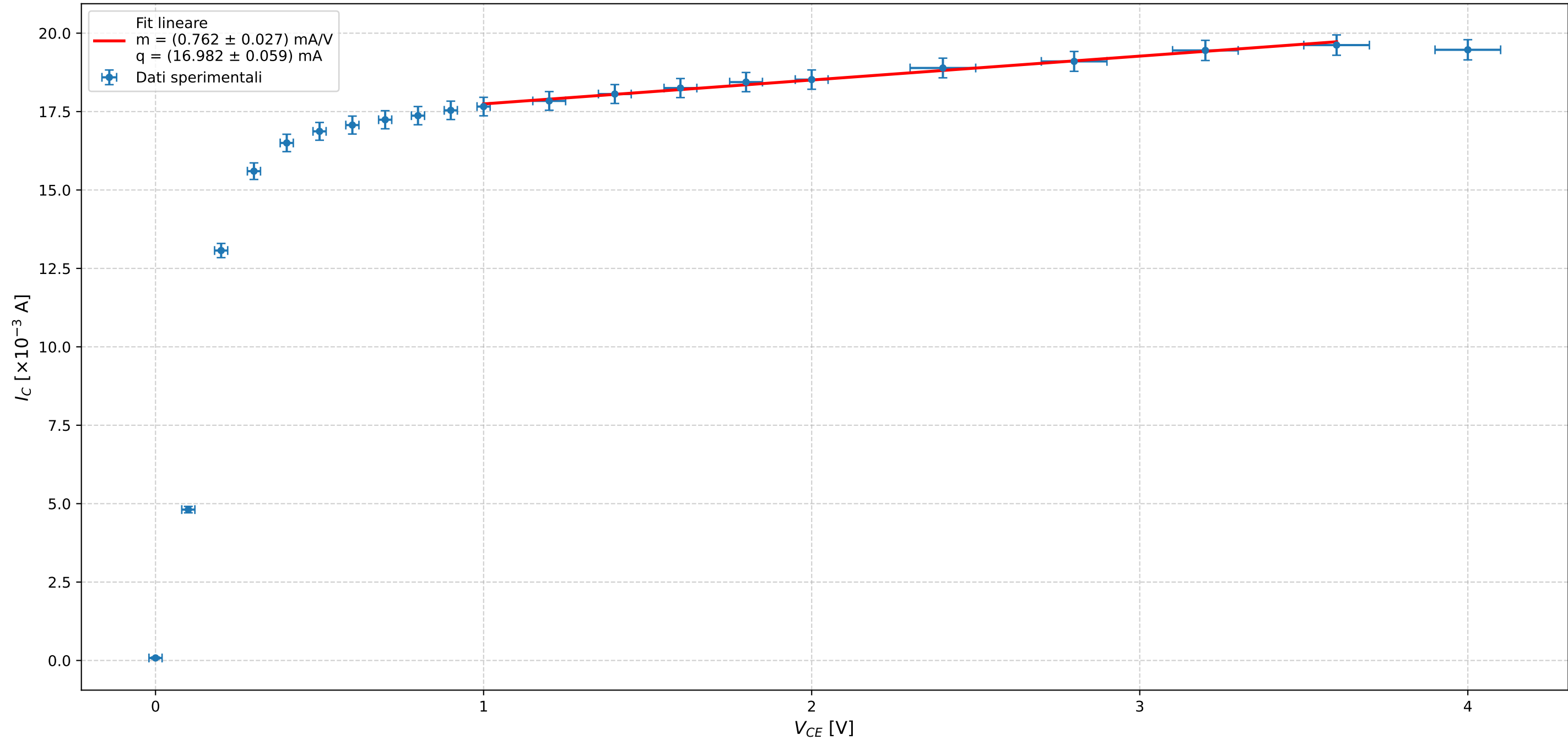
Caratteristica di uscita BJT PNP Configurazione a emettitore comune
