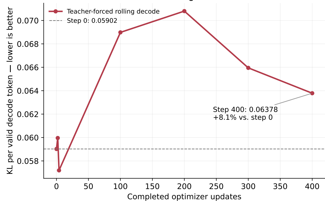
Held-out rolling decode KL
