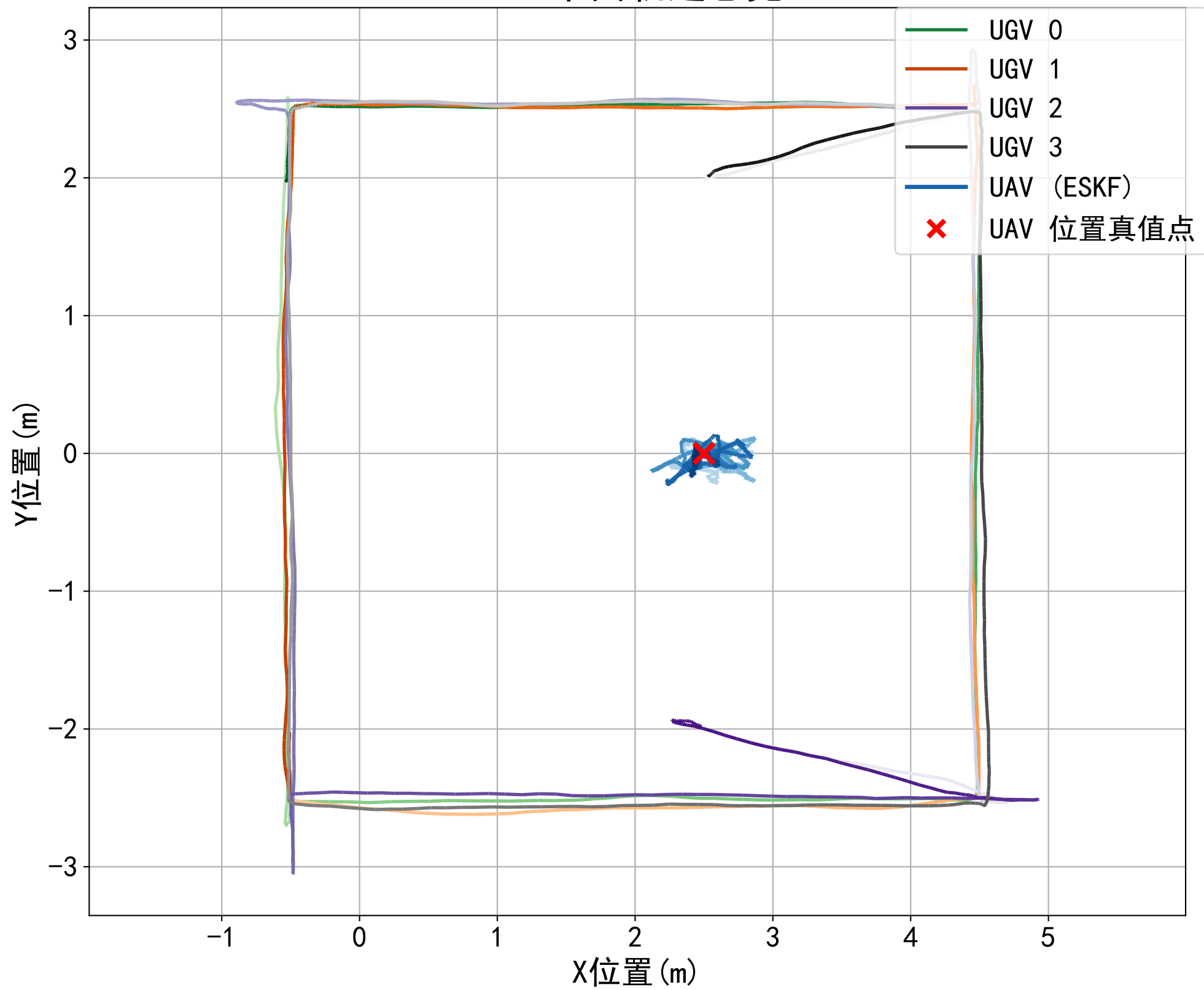
XY 平面轨迹总览
