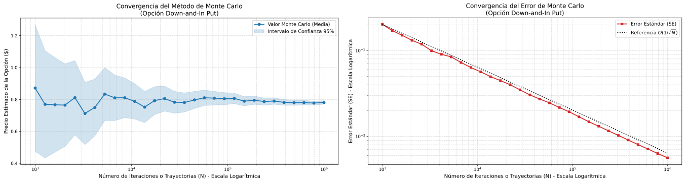
Figura 6.3: Convergencia estadística del método de Monte Carlo con algoritmo Longstaff-Schwartz. A la izquierda, evolución del precio estimado y estrechamiento del intervalo de confianza al 95% conforme crece el número de trayectorias M . A la derecha, caída del error estándar (SE) en escala logarítmica, confirmando un ajuste exacto a la tasa teórica asintótica O(1/\sqrt{M}) .
