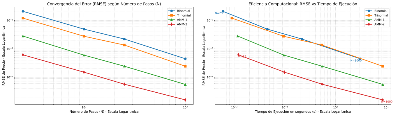
Figura 4.12: Convergencia del error y eficiencia computacional del AMM frente a modelos de red estándar. A la izquierda, evolución del RMSE en función del número de pasos temporales N (escala logarítmica). A la derecha, diagrama de eficiencia (RMSE vs. tiempo de ejecución en segundos), evidenciando que el AMM-2 alcanza un error inferior a 10^{-4} con un tiempo de cómputo sustancialmente menor al de un trinomial estándar de miles de pasos.
