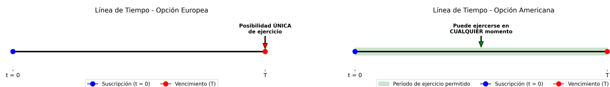
Figura 2.2: Comparación entre las líneas de tiempo de ejercicio de una opción europea (ejercicio exclusivo en t = T ) y una opción americana (ejercicio admisible en cualquier instante continuo t \in [0, T] ).
