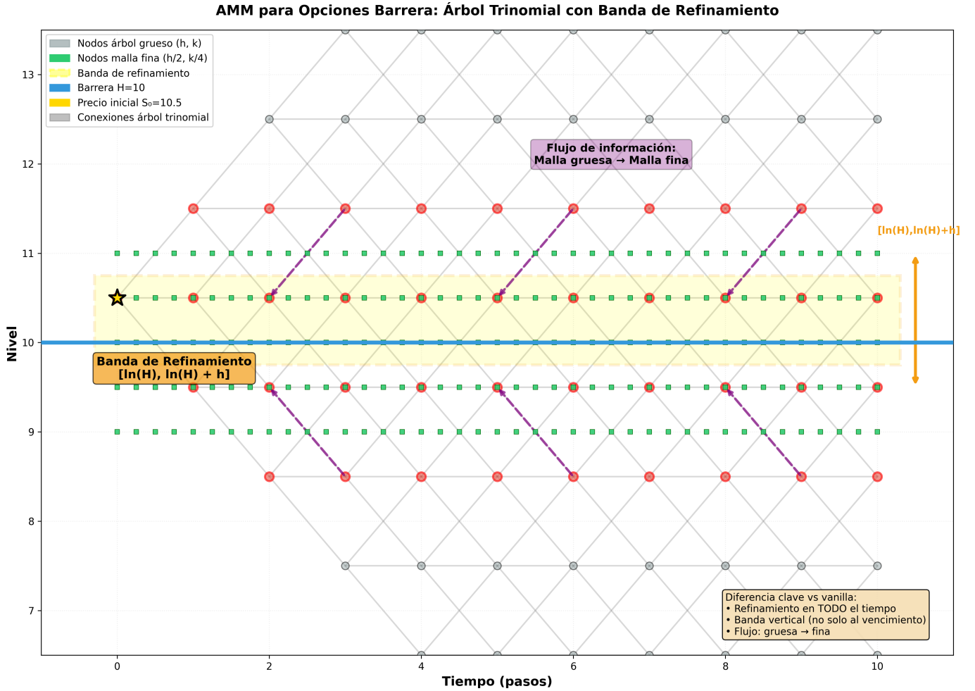
Figura 4.7: Estructura del AMM para opciones barrera. Se ilustra el árbol trinomial base con una banda vertical de malla fina a lo largo de toda la dimensión temporal. La malla fina se construye exclusivamente del lado activo de la barrera: para una opción down-and-out, la banda de refinamiento cubre el intervalo [\ln(H), \ln(H) + h] en el espacio logarítmico, es decir, desde la barrera H hasta el primer nodo grueso por encima de ella. Se muestra el precio inicial S_0 cerca de H para evidenciar la solución al problema del límite. Las flechas indican el flujo de información (condiciones de borde) que se transfiere desde la malla gruesa hacia la malla fina para la valoración.
