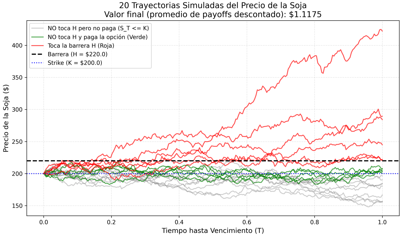
Figura 6.1: Muestra de 20 trayectorias simuladas para una opción Call Up-and-Out sobre el precio de la soja ( S_0 = \$200, K = \$200, H = \$220, T = 1 ). Las líneas rojas representan trayectorias que tocan la barrera H , quedando invalidadas con valor cero. Las líneas verdes corresponden a trayectorias que permanecen por debajo de H y expiran en zona de ganancia ( S_T > K ). Las líneas grises expiran sin valor. El precio de la opción se estima como el promedio descontado de los pagos terminales válidos.
