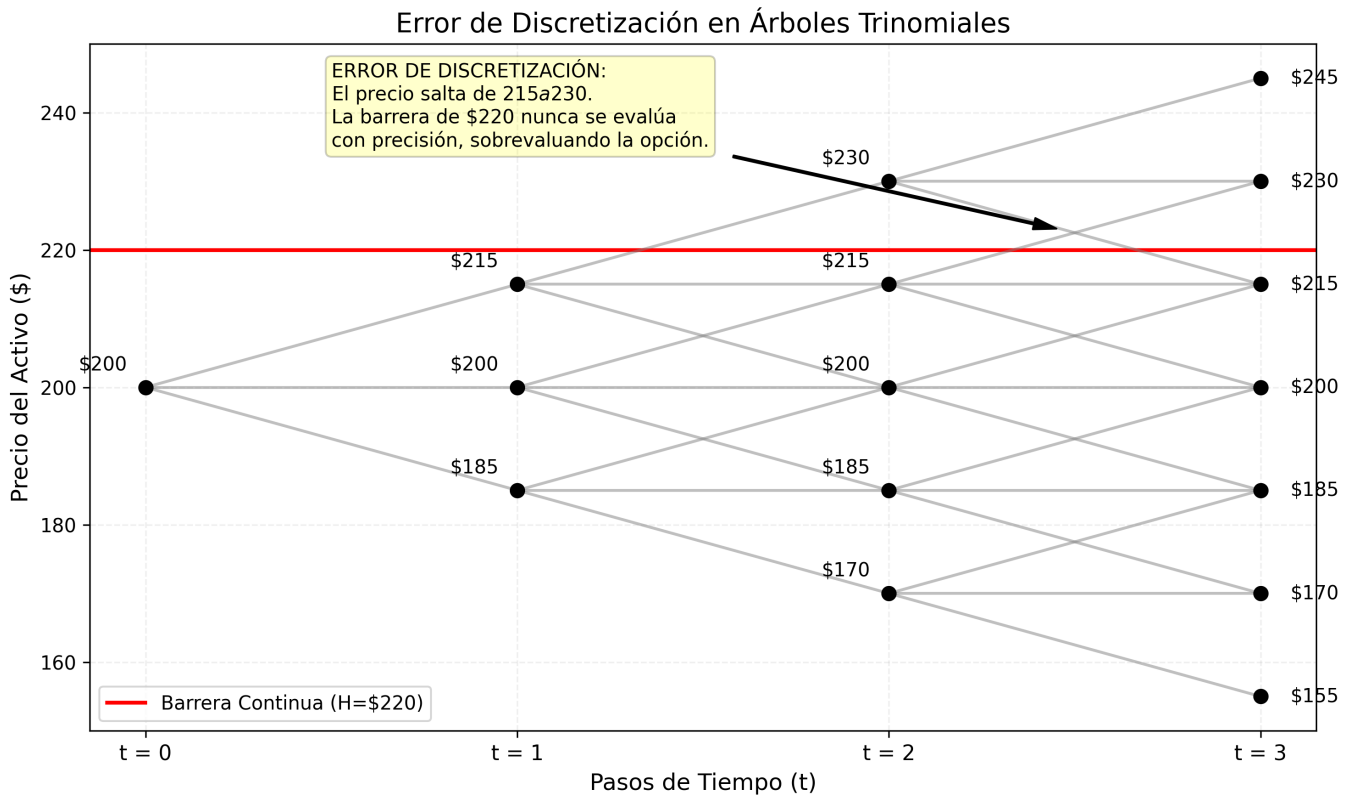
Figura 4.3: Error de discretización geométrica en un árbol trinomial estándar cuando la barrera continua ( H = \$220 ) no coincide con una capa de nodos discretos. El salto abrupto entre $215 y $230 distorsiona la detección del evento de barrera.
