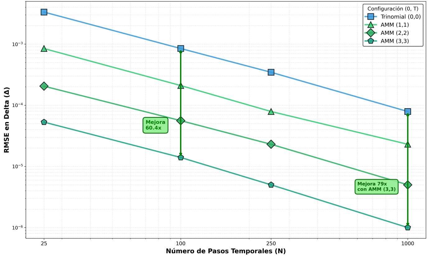
Figura 4.10: Precisión en el cálculo de Delta mediante ramificación cuadrinomial. Se compara el RMSE en Delta para diferentes configuraciones AMM (0, T) , donde 0 es el inicio de la opción y T es el final de la misma. La ramificación cuadrinomial permite calcular Delta mediante diferencias finitas. AMM (3,3) logra una mejora de 60x vs Trinomial en N=100 , con un incremento de tiempo < 3\% . Notablemente, AMM (1,0) mejora Delta sin costo adicional al refinar solo la región crítica.
