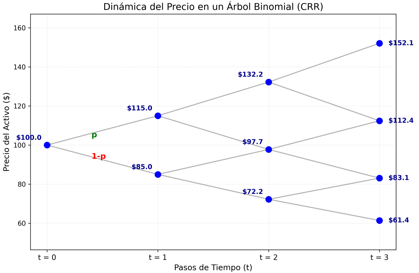
Figura 4.1: Evolución del precio de un activo en un árbol binomial recombinante de Cox, Ross y Rubinstein (CRR) a tres pasos temporales ( t = 0, 1, 2, 3 ). En cada nodo, el precio puede ascender con probabilidad p o descender con probabilidad 1 - p .
