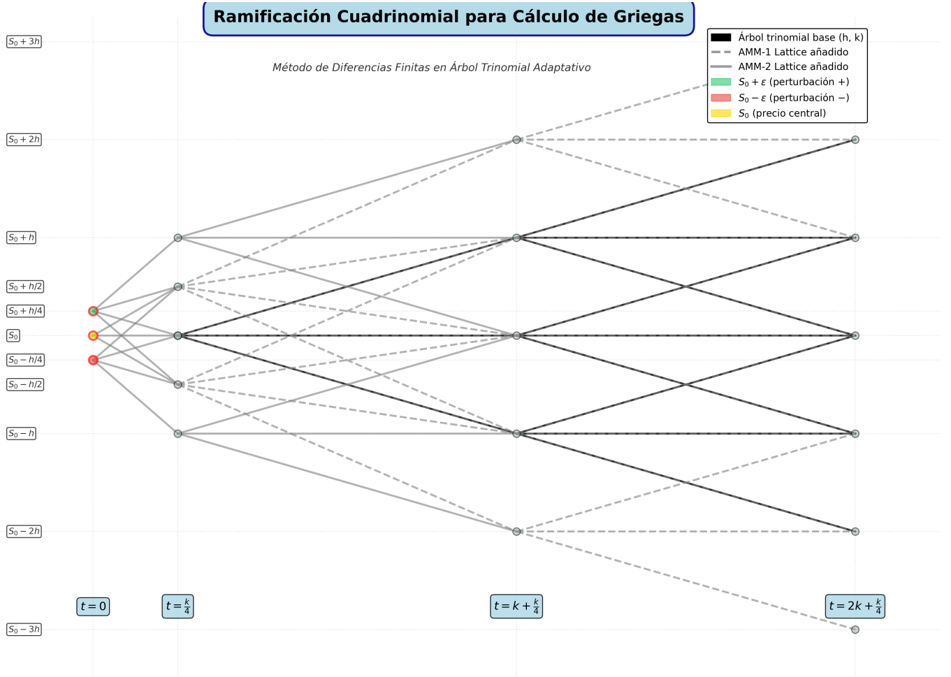
Figura 4.9: Ramificación cuadrinomial para el cálculo de griegas mediante diferencias finitas. Se muestra un árbol trinomial base (nodos grises, conexiones negras gruesas) con nodos adicionales en t = 0 ubicados en S_0 + \epsilon (verde) y S_0 - \epsilon (rojo), donde \epsilon = h/4 es una perturbación pequeña. Las líneas sólidas grises representan ramificación cuadrinomial (4 ramas) desde los nodos perturbados y los nodos extremos en t = k/4 , permitiendo calcular simultáneamente Delta y Gamma con alta precisión.
