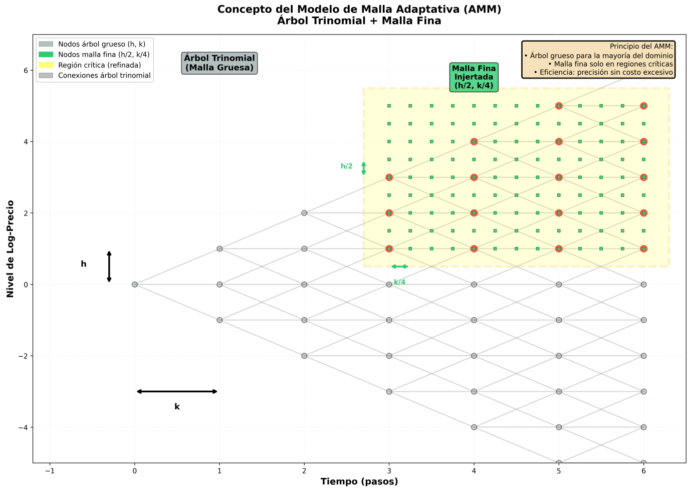
Figura 4.6: Concepto del Modelo de Malla Adaptativa (AMM). Se muestra un árbol trinomial base (nodos grises) que constituye la malla gruesa. Sobre este se injerta una malla fina (cuadrados verdes) con pasos reducidos en la región crítica. La operación transfiere los valores del árbol grueso hacia los bordes del árbol fino, para luego resolver la valoración internamente.
