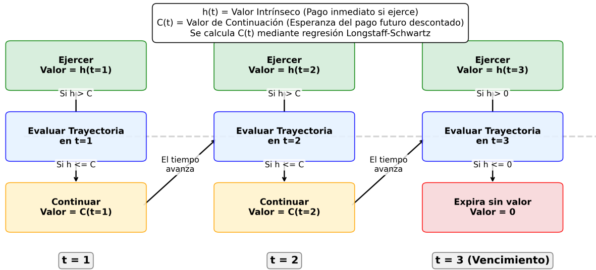
Diagrama de Decisión: Método Longstaff-Schwartz
