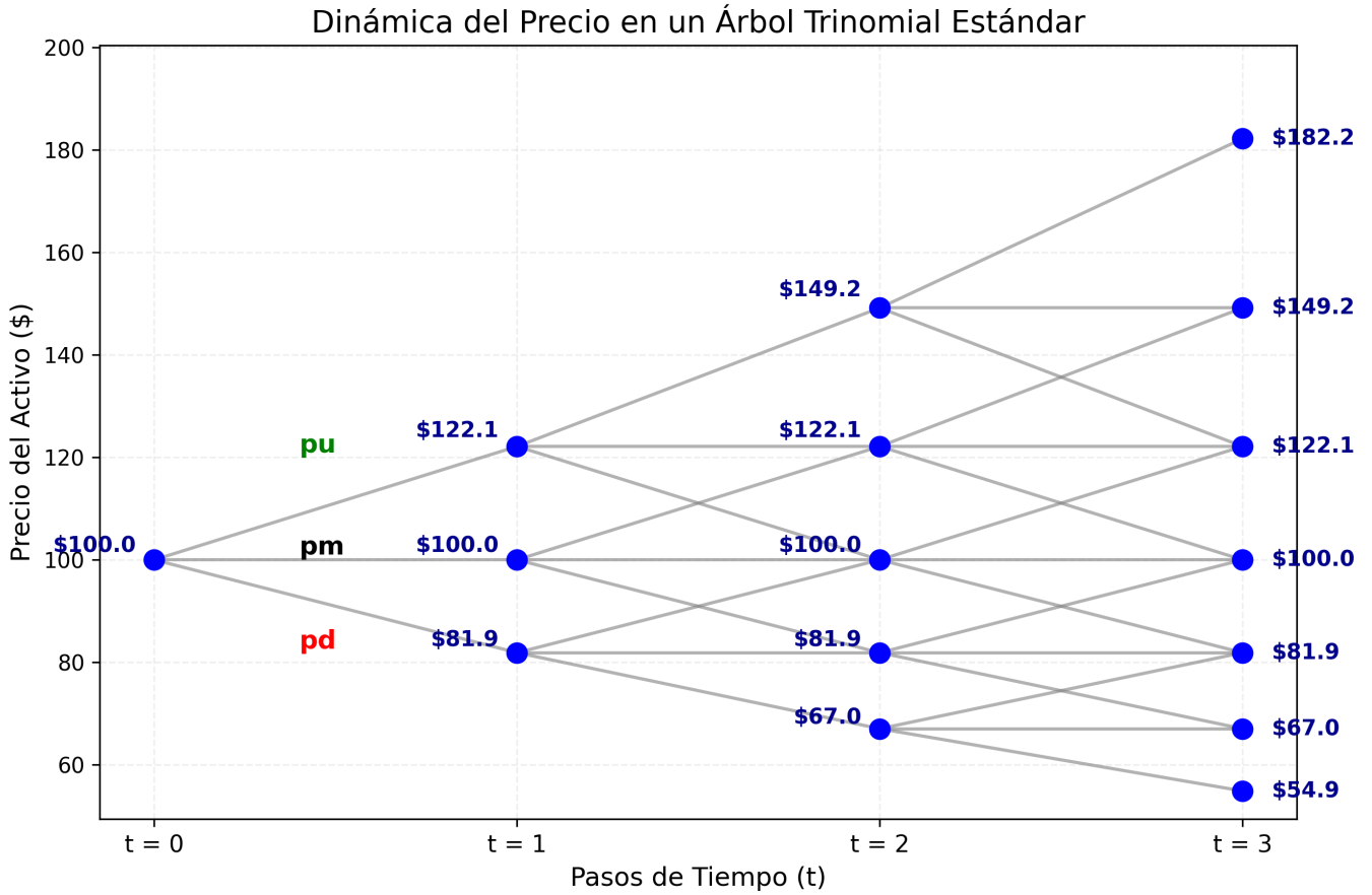
Figura 4.2: Estructura de ramificación y dinámica de precios en un árbol trinomial estándar recombinante a tres pasos temporales. Desde cada nodo se despliegan tres trayectorias alternativas ( u , m , d ) ponderadas por sus respectivas probabilidades neutrales al riesgo ( p_u, p_m, p_d ).
