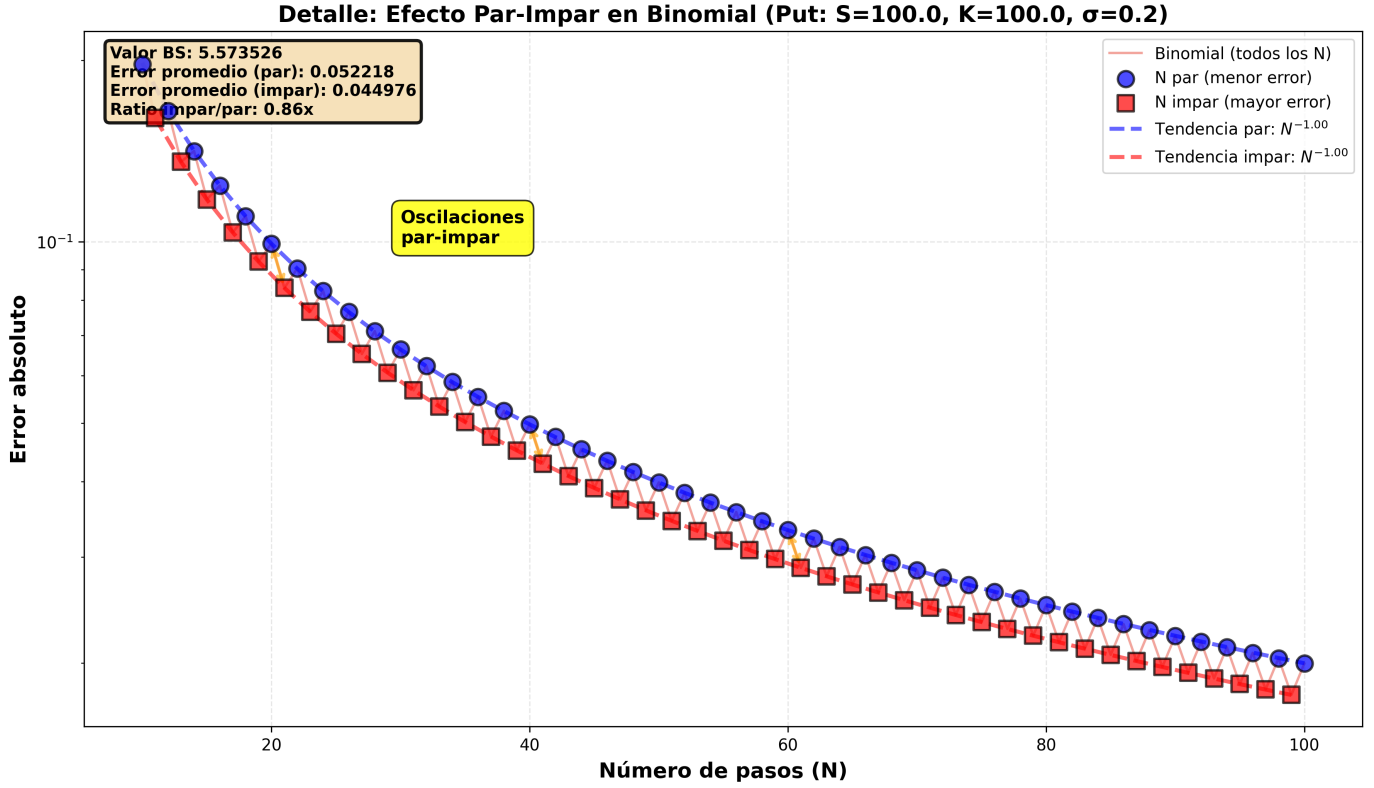
Figura 4.5: Ejemplo de convergencia inestable causada por el error de no linealidad. Históricamente, el efecto “par-impar” en modelos binomiales demostraba cómo la falta de alineación de los nodos finales generaba oscilaciones. El AMM elimina completamente estos problemas de no linealidad en las estructuras trinomiales.
