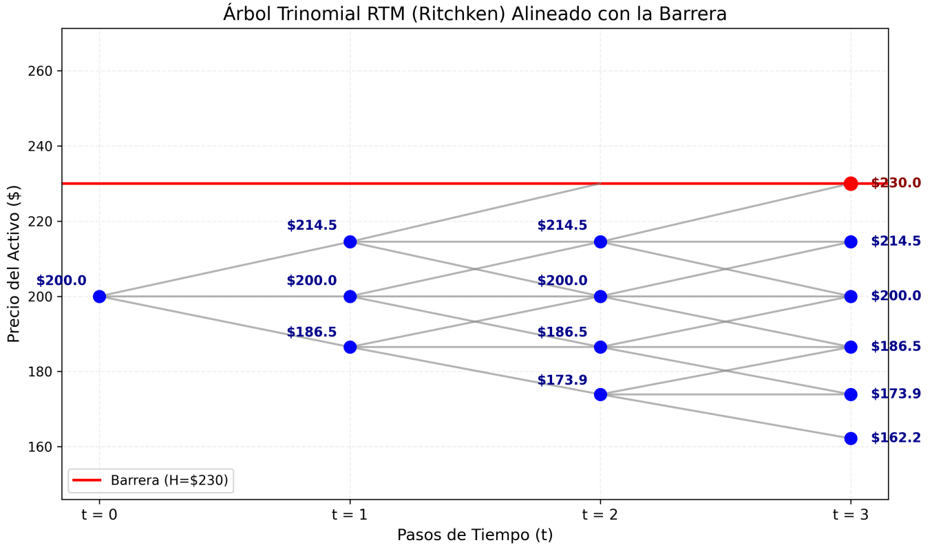
Figura 4.4: Árbol Trinomial Restringido forzado a alinear una capa horizontal de nodos directamente sobre la barrera H = \$230 . Aunque previene el sesgo de poda en la frontera roja, sufre una severa explosión de complejidad temporal si S_0 se sitúa a poca distancia de H .
