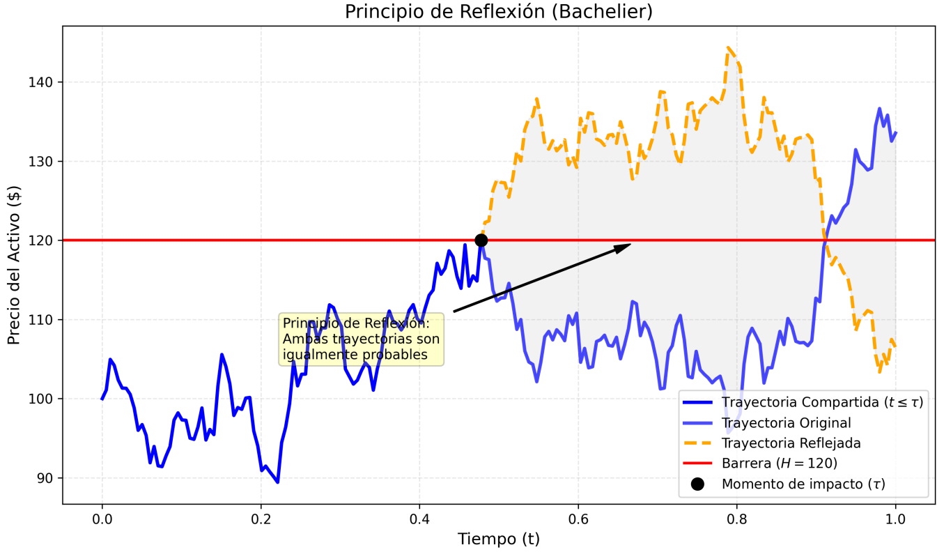
Figura 3.1: Principio de Reflexión de Bachelier aplicado a la valoración de opciones barrera. Para cualquier trayectoria que impacta la barrera H en el instante de primer pasaje \tau y finaliza en un nivel dado, existe una trayectoria simétrica (reflejada) que posee idéntica probabilidad estadística bajo el Movimiento Browniano. Esta equivalencia geométrica permite descomponer la probabilidad de cruce en términos de la función de distribución normal estándar acumulada N(\cdot) .
