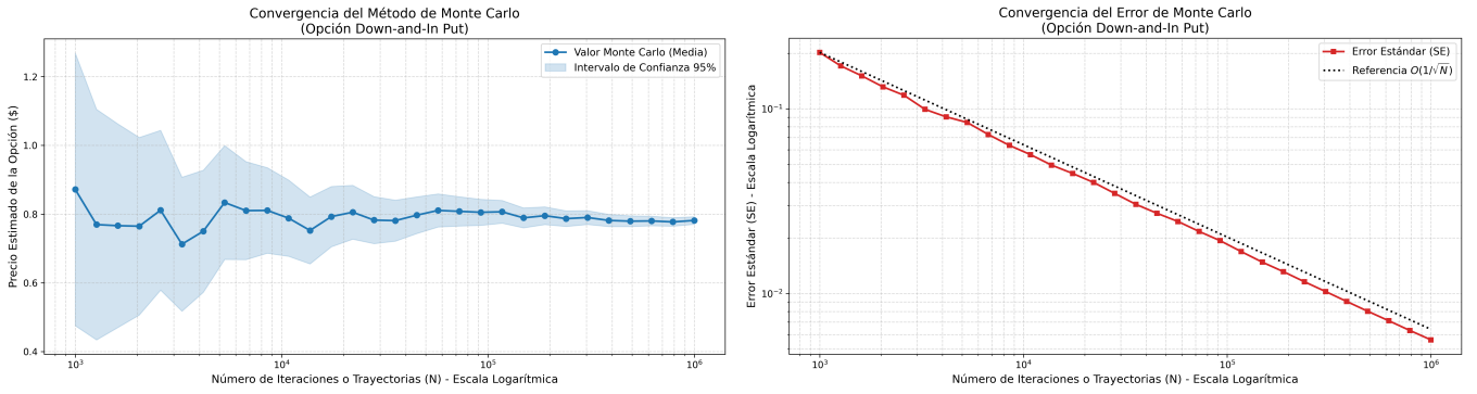
Figura 6.3: Convergencia estadística del método de Monte Carlo con algoritmo Longstaff-Schwartz. A la izquierda, evolución del precio estimado y estrechamiento del intervalo de confianza al 95% conforme crece el número de trayectorias M . A la derecha, caída del error estándar (SE) en escala logarítmica, confirmando un ajuste exacto a la tasa teórica asintótica O(1/\sqrt{M}) .
