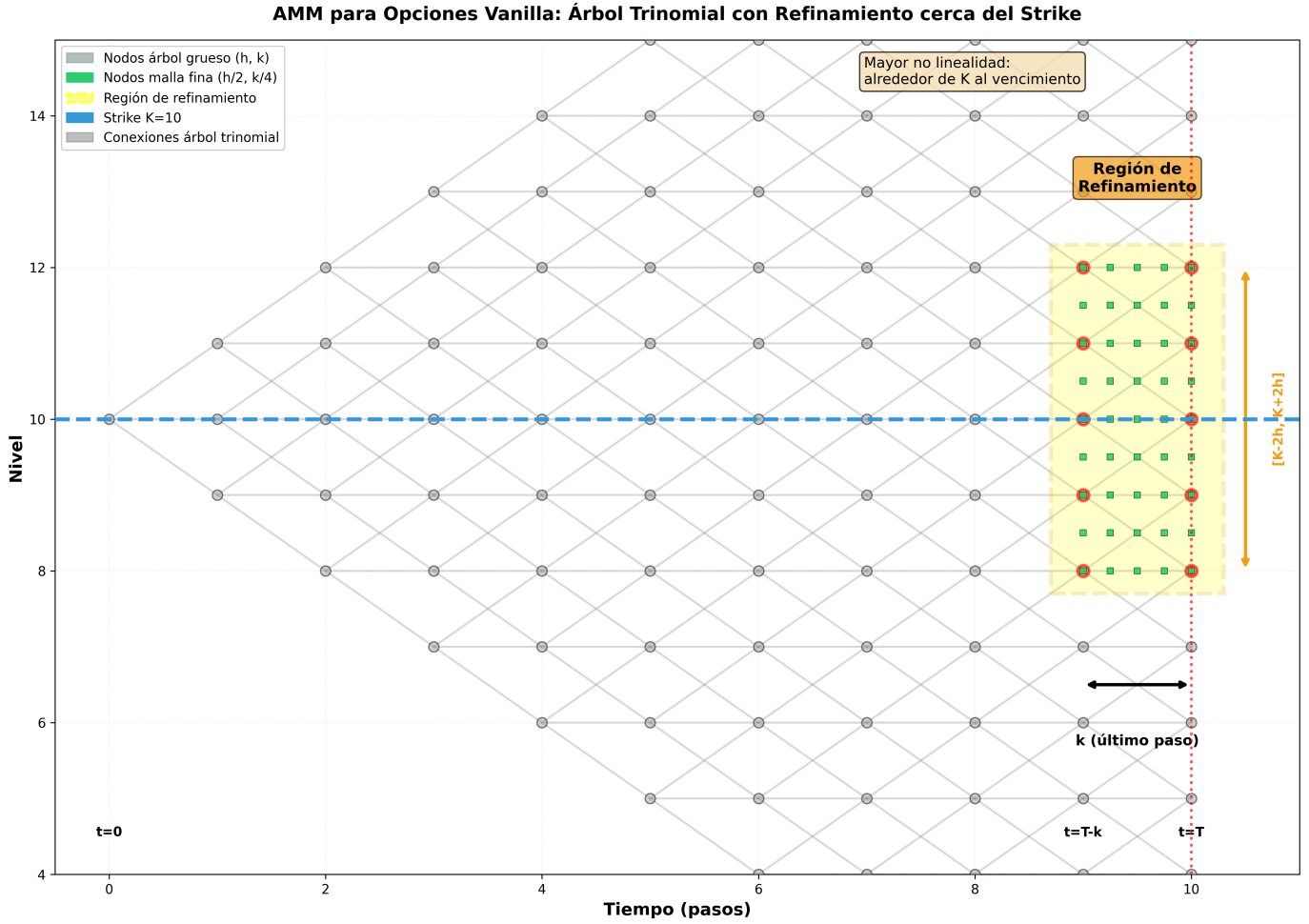
Figura 4.8: Estructura del AMM para opciones vanilla. Se muestra un árbol trinomial (nodos grises con conexiones grises) que constituye la malla gruesa. Sobre este árbol se inserta una malla fina (cuadrados verdes pequeños) con pasos h/2 y k/4 únicamente en la región crítica (rectángulo amarillo): temporal [T-k, T] y espacial [K-2h, K+2h] . La línea azul punteada marca el strike K donde ocurre la mayor no linealidad al vencimiento. Esta estrategia concentra la resolución donde más se necesita: alrededor del precio de ejercicio al vencimiento.
