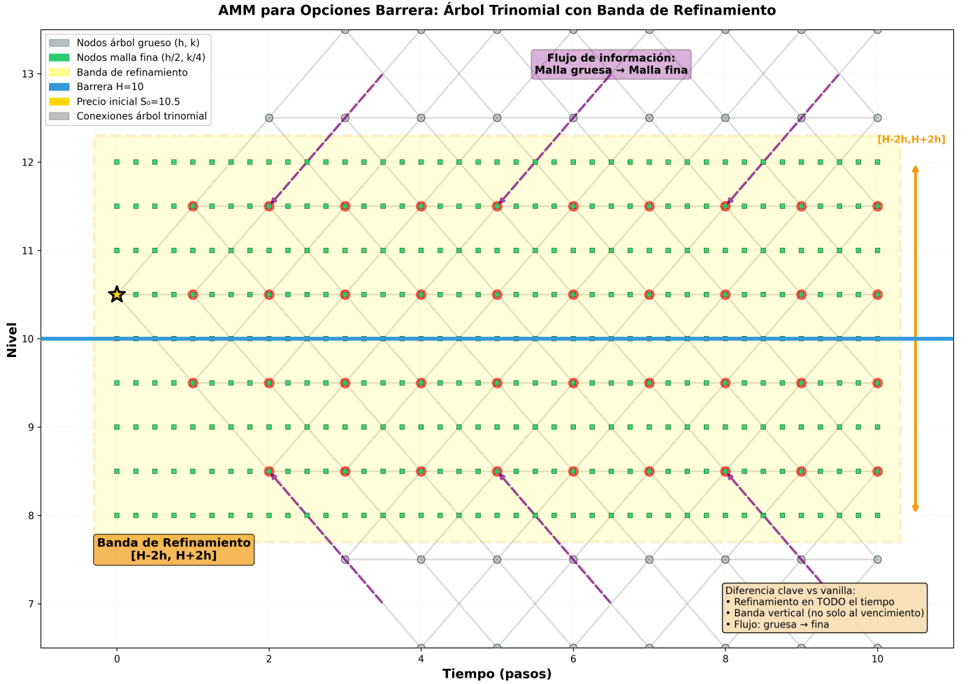
Figura 4.4: Estructura del AMM para opciones barrera. Se ilustra el árbol trinomial base con una banda vertical de malla fina a lo largo de toda la dimensión temporal, centrada en la barrera H . La región de refinamiento está delimitada por [H - 2h, H + 2h] . Se muestra el precio inicial S_0 cerca de H para evidenciar la solución al problema del límite. Las flechas indican el flujo de información (condiciones de borde) que se transfiere desde la malla gruesa hacia la malla fina para la valoración.
