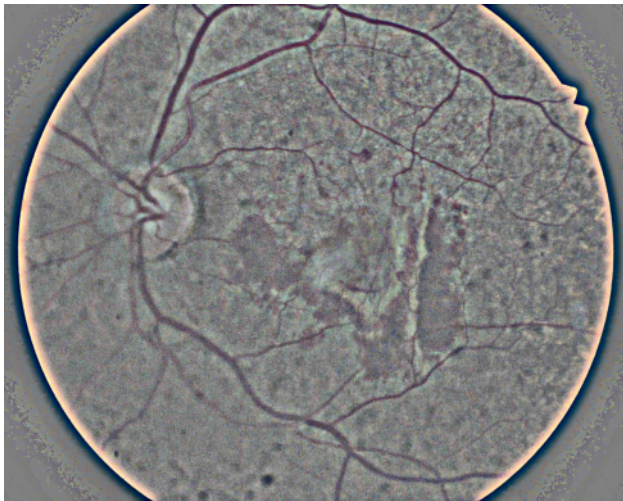
Step 4: CLAHE
