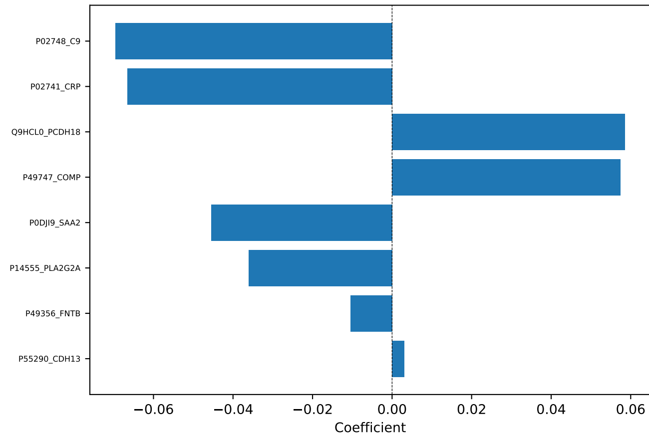
LASSO (8 features)
