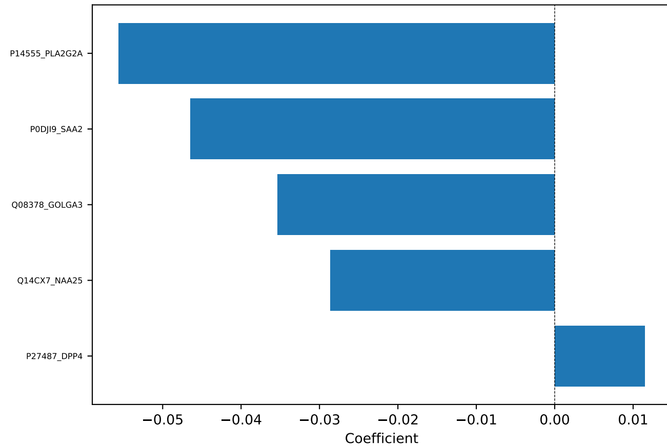
LASSO (5 features)
