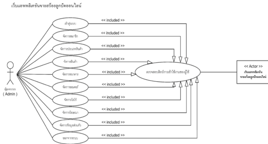
รูปที่ 3.2 Use Case Diagram แอปพลิเคชันขายสร้อยลูกปัดออนไลน์
