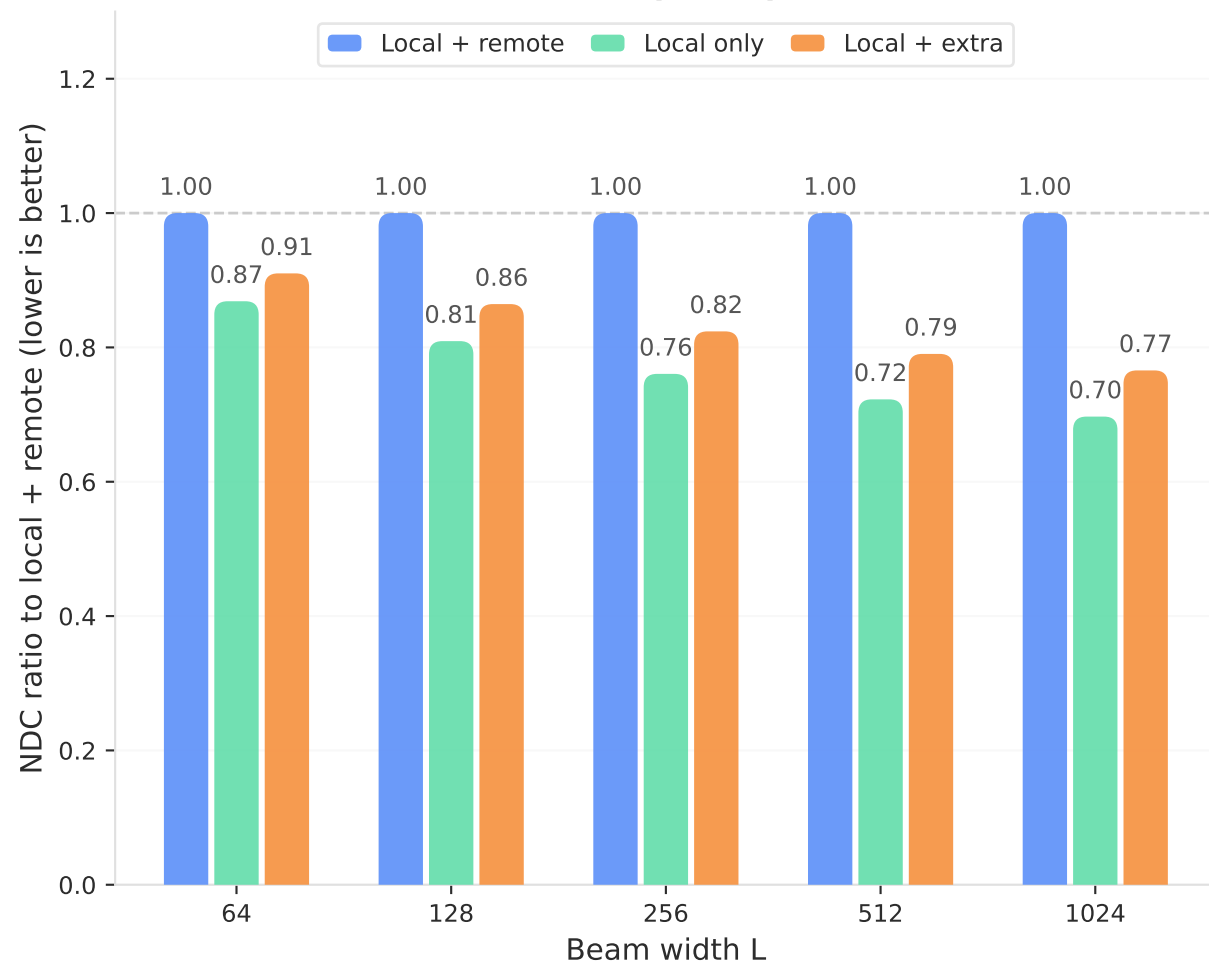
SIFT (k=10)
