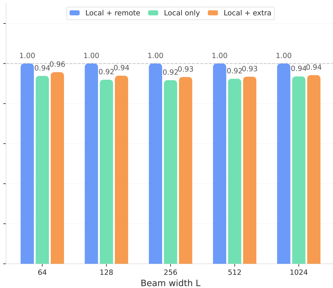
GIST (k=10)
