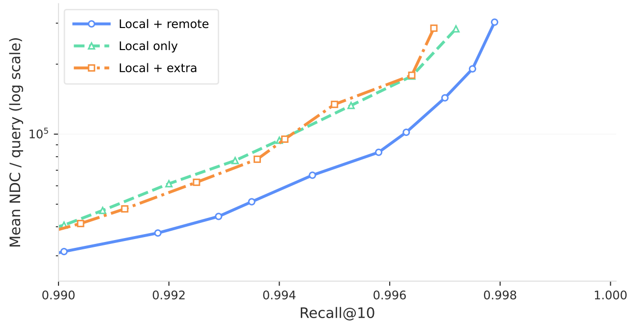
GIST (k=10)
