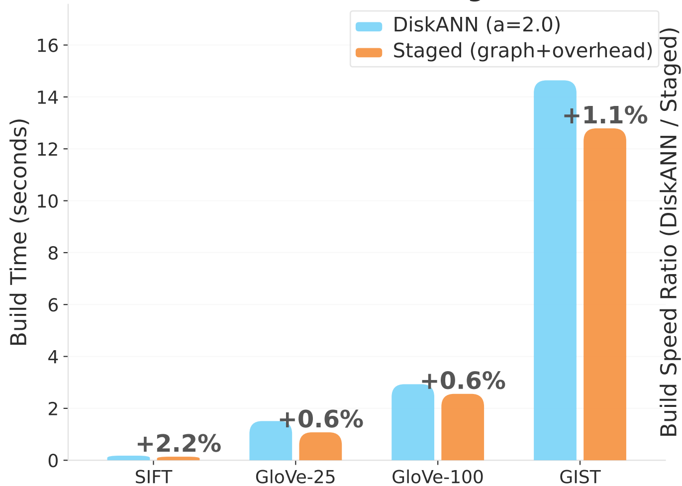
Build Time: DiskANN vs StagedDiskANN
