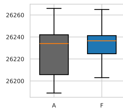
LND
