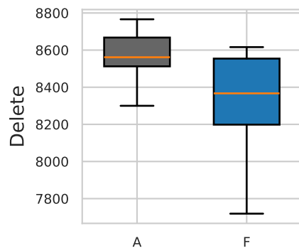
CLN
