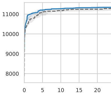
ECLAIR
