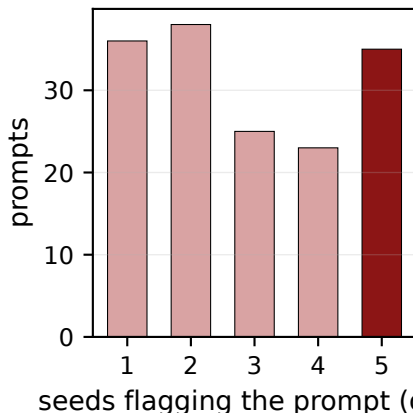
(b) Per-prompt flag count
