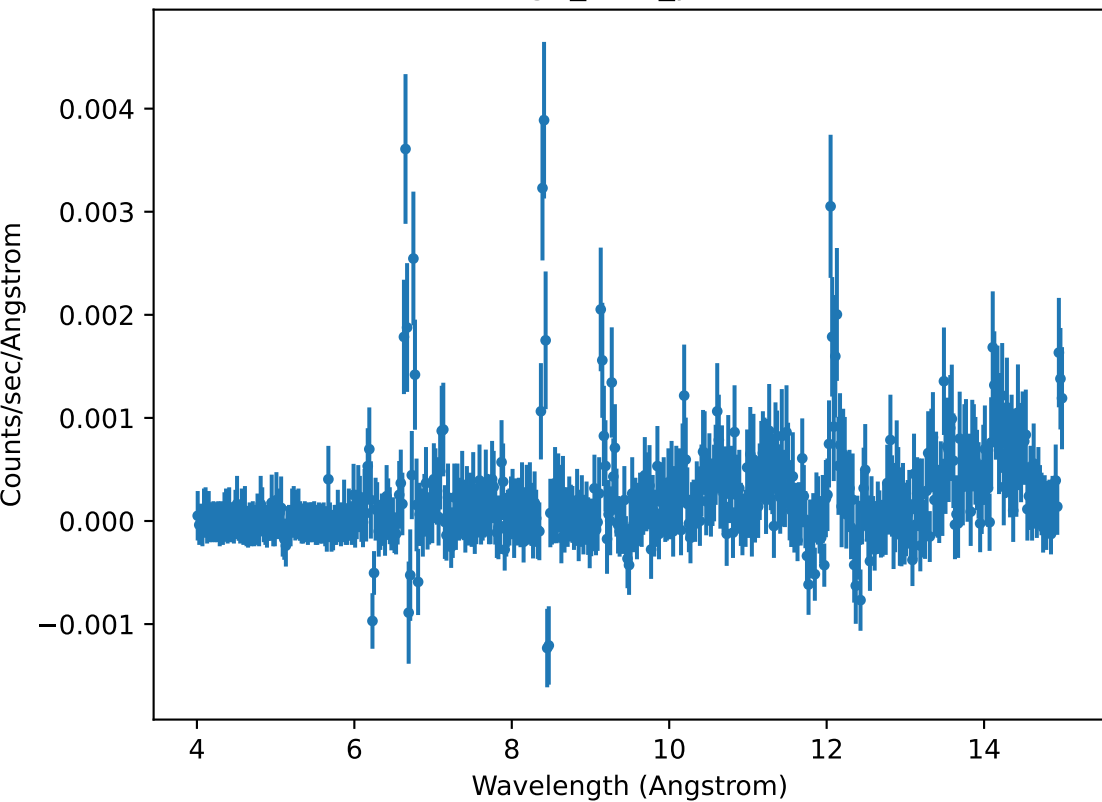
EQPegB_both pha2.fits
