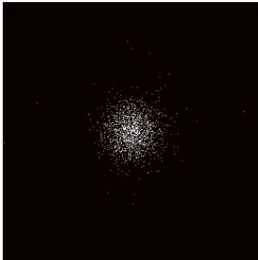
diffuse_evt2.fits
