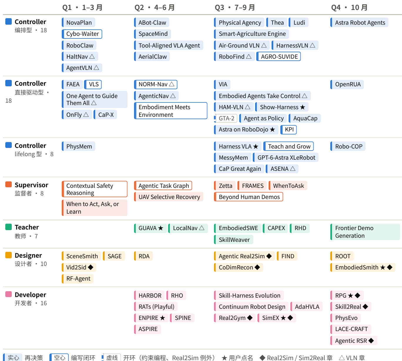
图6 2026年论文按 Seat 与季度分布。 下半年明显加速；Developer 和 lifelong 型 Controller 几乎都出现在 Q3 以后，对应 coding agent 和 harness 进化的浪潮。
