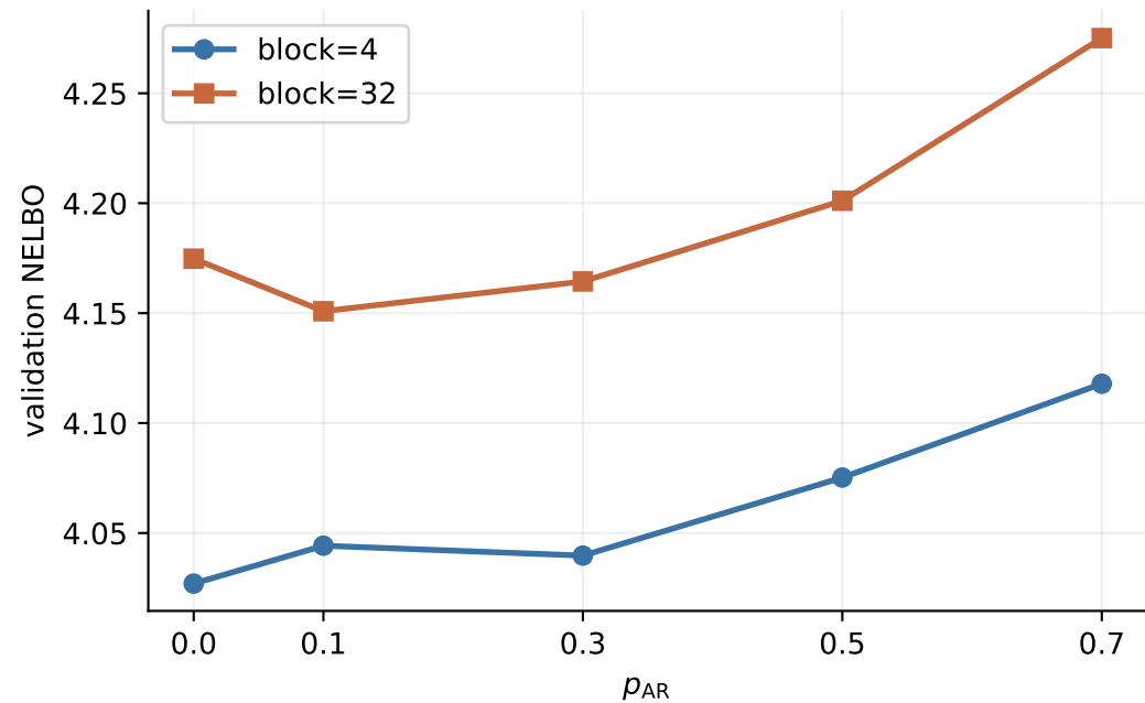
Validation diffusion NELBO
