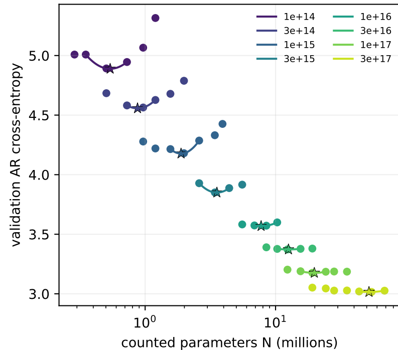
Pure autoregressive IsoFLOP profiles
