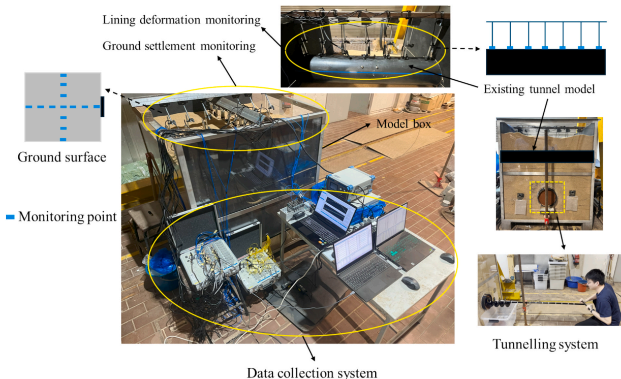
Fig. 6. Test apparatus.
