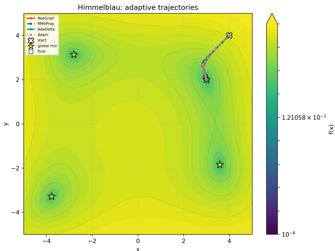
Рис. 42: Himmelblau, x_0 = (4.0, 4.0) : адаптивные методы
