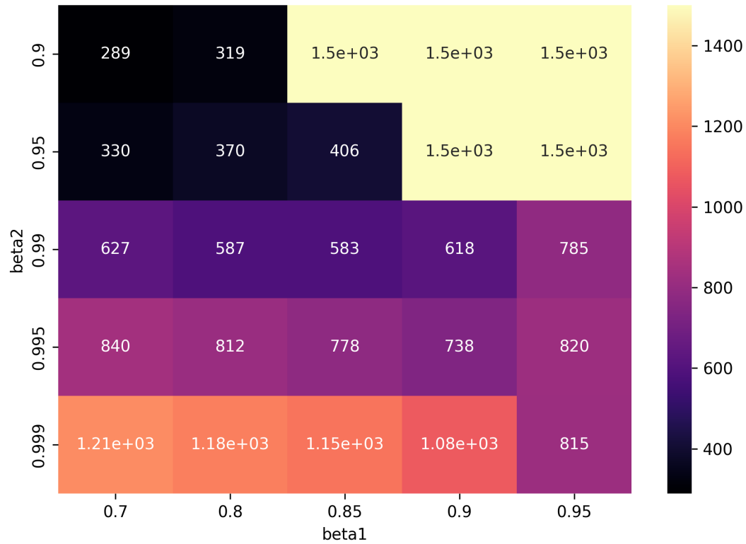
Рис. 8: Adam: чувствительность к \beta_1 и \beta_2 на хорошо обусловленной функции
