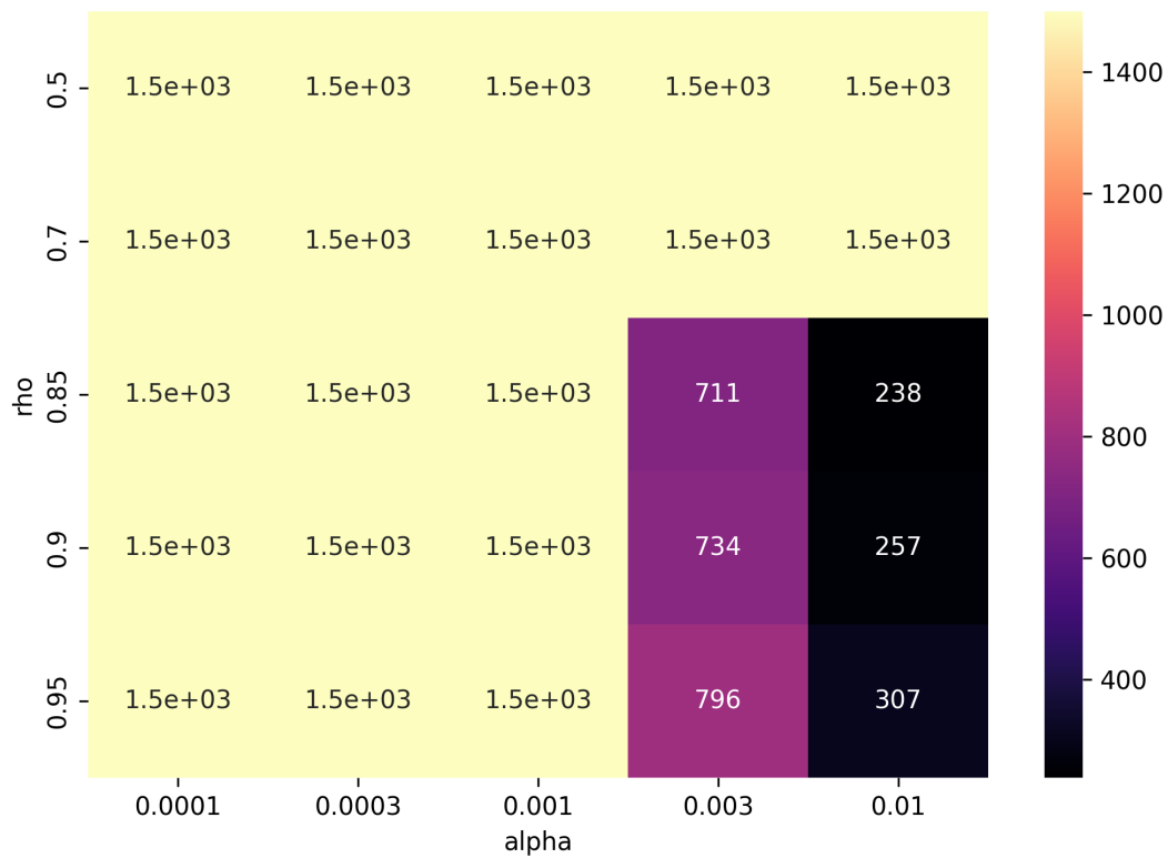
Рис. 5: RMSProp: чувствительность к \alpha и \rho на хорошо обусловленной функции
