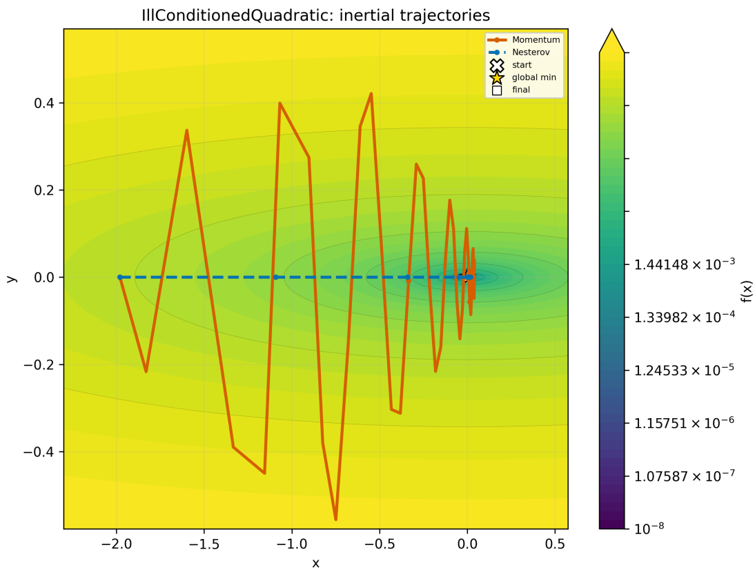
Рис. 21: Инерционные методы на плохо обусловленной квадратичной функции
