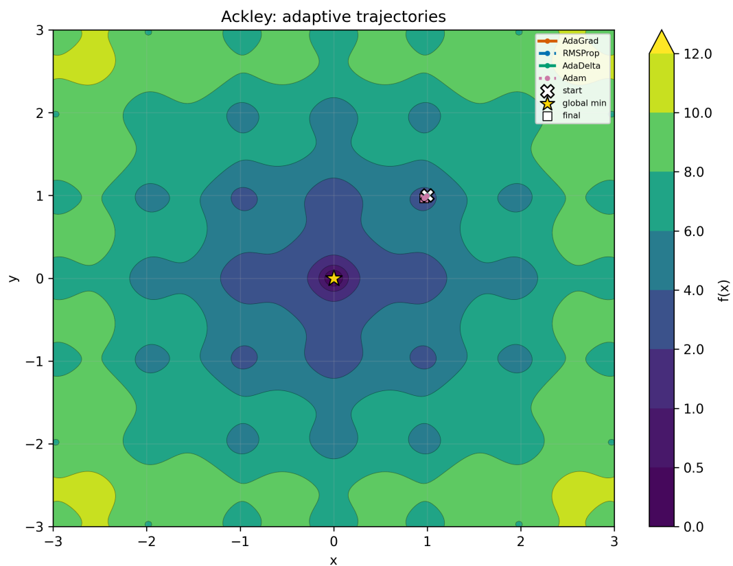
Рис. 32: Ackley, x_0 = (1.0, 1.0) : адаптивные методы
