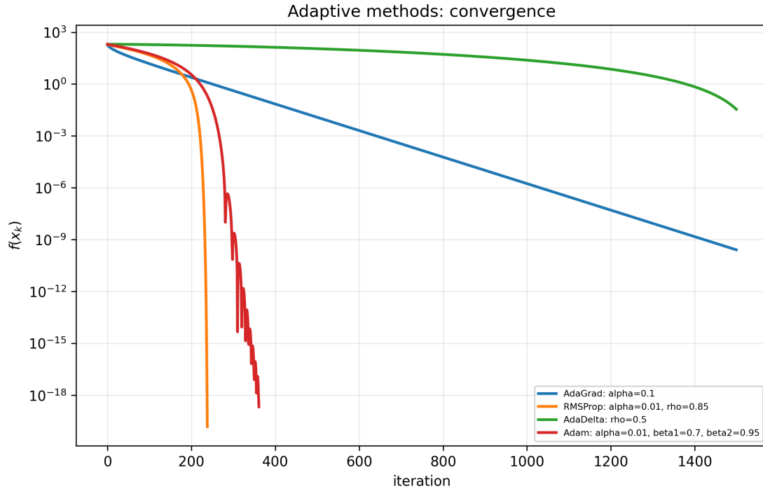
Рис. 24: Адаптивные методы: сходимость f(x_k) на плохо обусловленной функции
