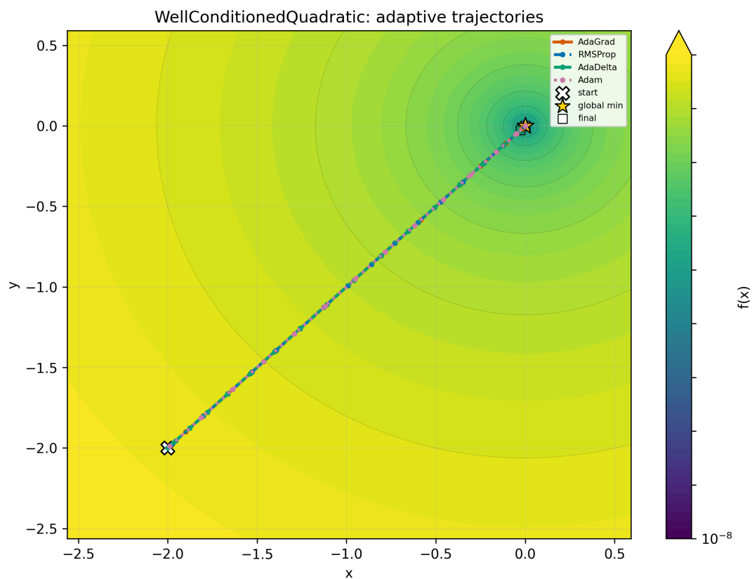
Рис. 18: Адаптивные методы на хорошо обусловленной квадратичной функции
