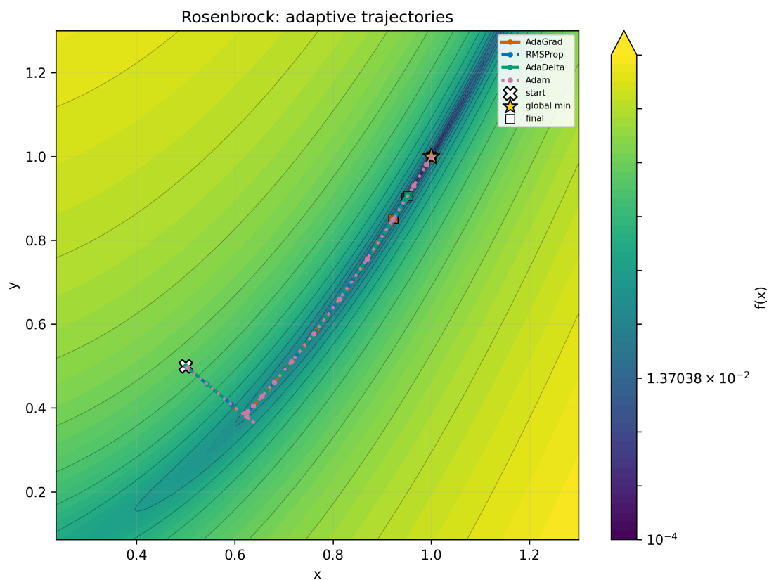
Рис. 30: Rosenbrock, x_0 = (0.5, 0.5) : адаптивные методы
