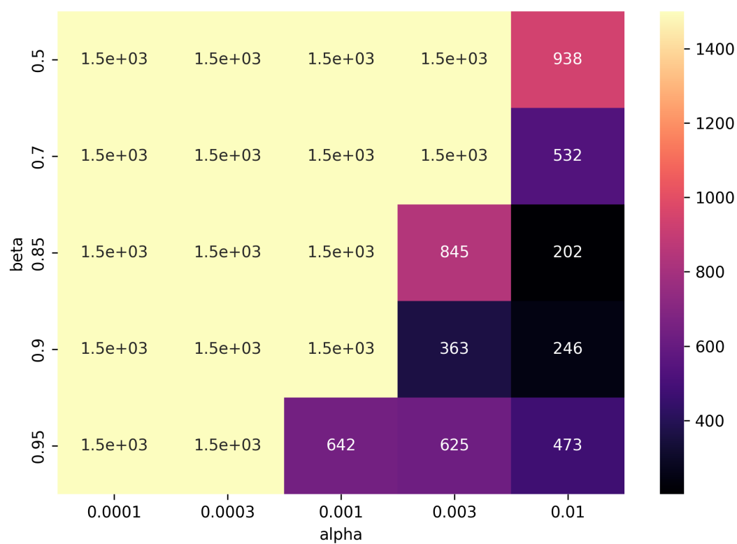
Рис. 10: Nesterov: чувствительность к \alpha и \beta на плохо обусловленной функции
