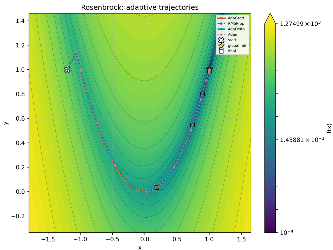
Рис. 26: Rosenbrock, x_0 = (-1.2, 1.0) : адаптивные методы
