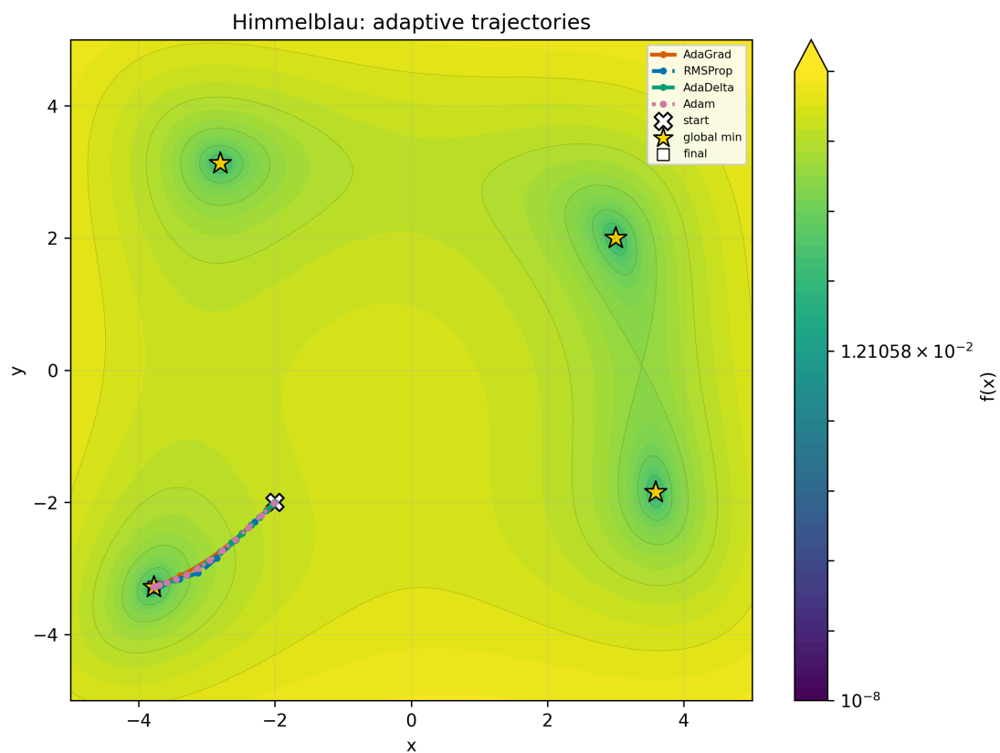
Рис. 40: Himmelblau, x_0 = (-2.0, -2.0) : адаптивные методы
