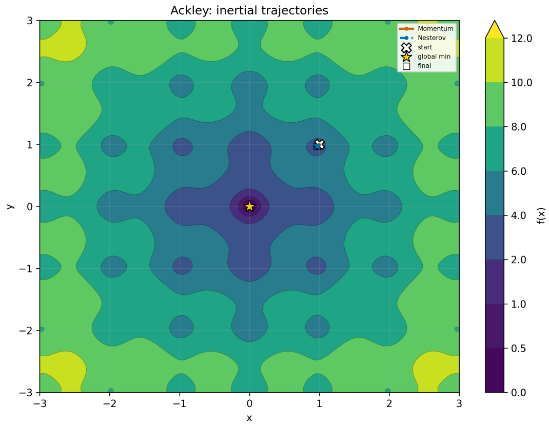
Рис. 31: Ackley, x_0 = (1.0, 1.0) : инерционные методы
