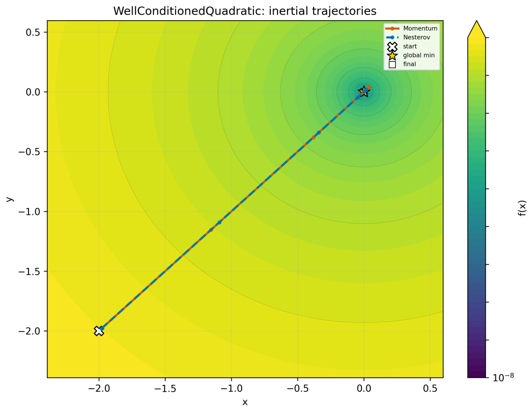
Рис. 17: Инерционные методы на хорошо обусловленной квадратичной функции
