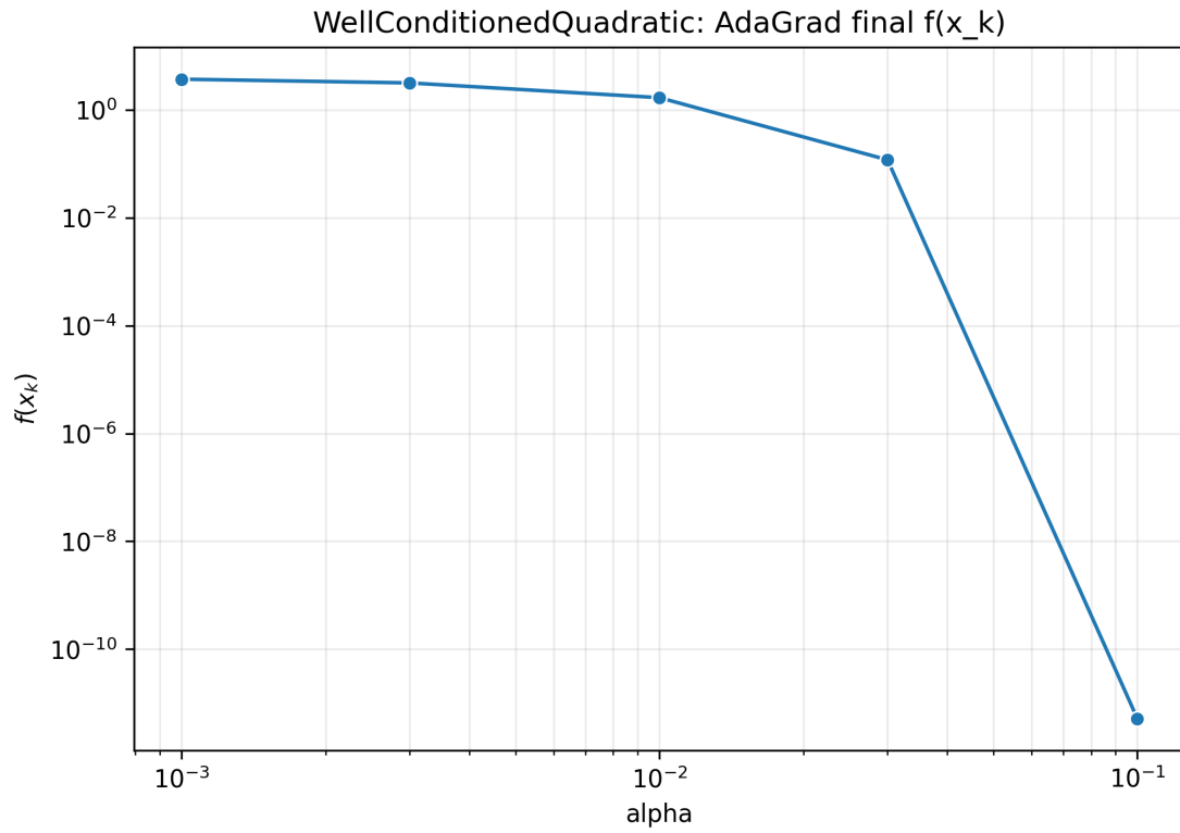
Рис. 4: AdaGrad: конечное значение f(x_k) при разных \alpha на хорошо обусловленной функции
