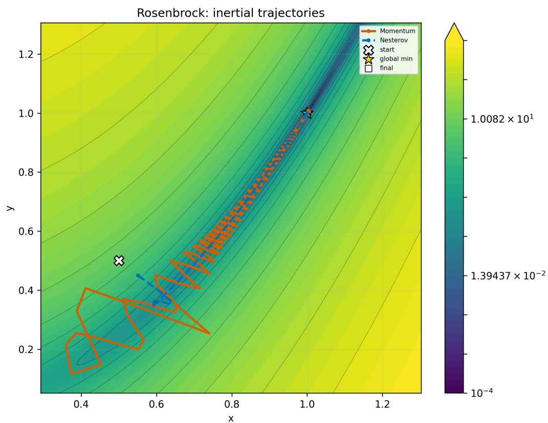
Рис. 29: Rosenbrock, x_0 = (0.5, 0.5) : инерционные методы
