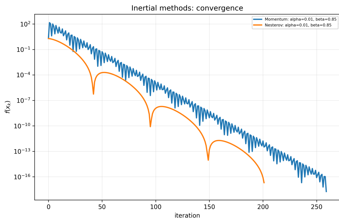
Рис. 23: Инерционные методы: сходимость f(x_k) на плохо обусловленной функции
