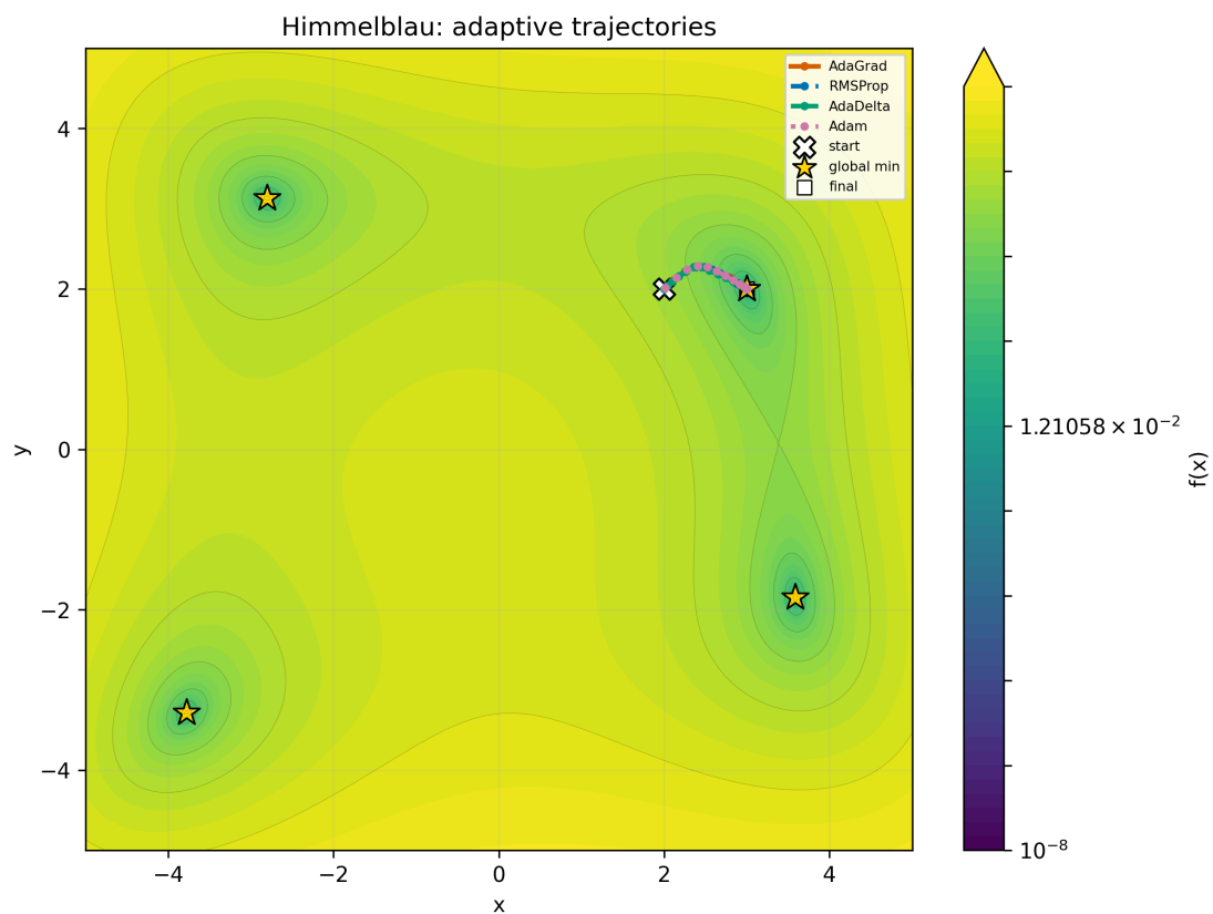
Рис. 38: Himmelblau, x_0 = (2.0, 2.0) : адаптивные методы
