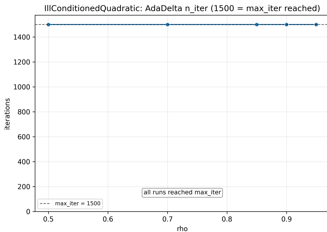
Рис. 14: AdaDelta: чувствительность к \rho на плохо обусловленной функции
