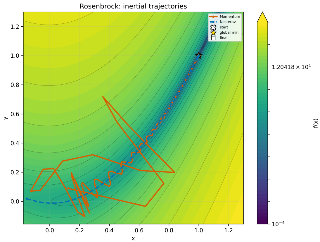
Рис. 25: Rosenbrock, x_0 = (-1.2, 1.0) : инерционные методы
