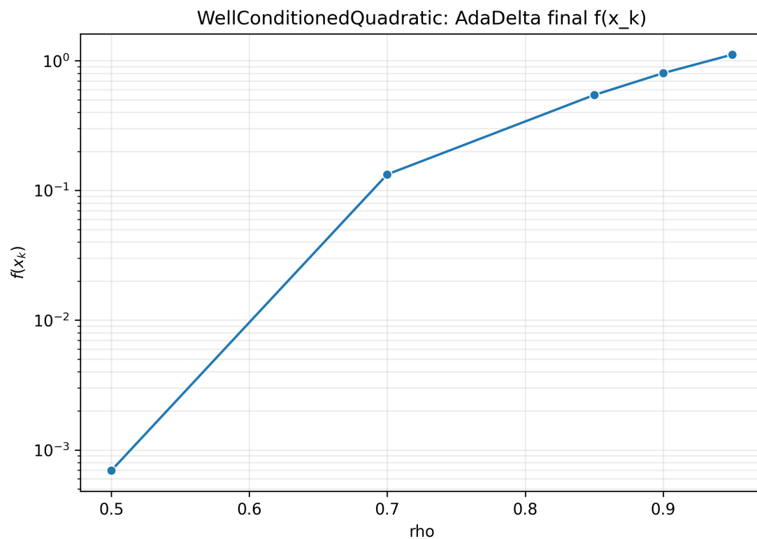
Рис. 7: AdaDelta: конечное значение f(x_k) при разных \rho на хорошо обусловленной функции
