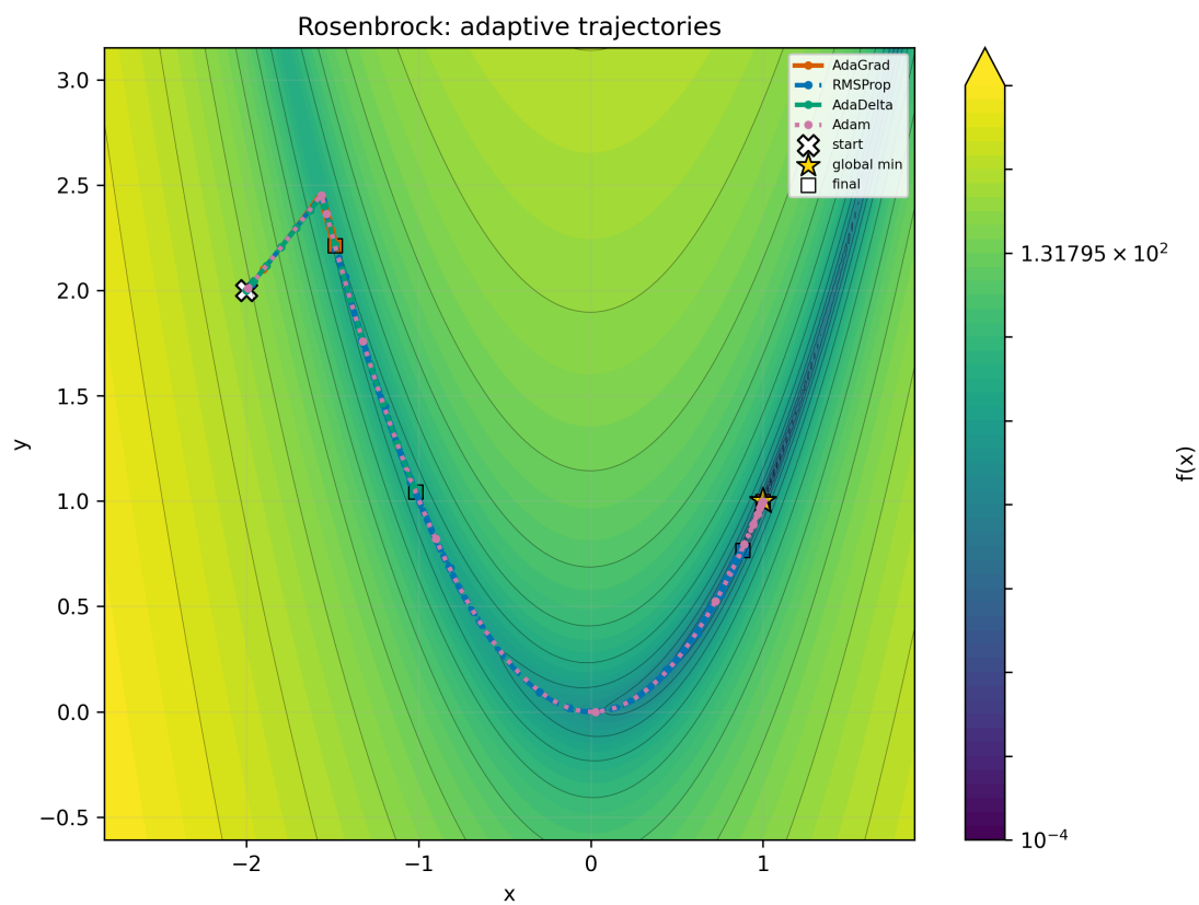
Рис. 28: Rosenbrock, x_0 = (-2.0, 2.0) : адаптивные методы
