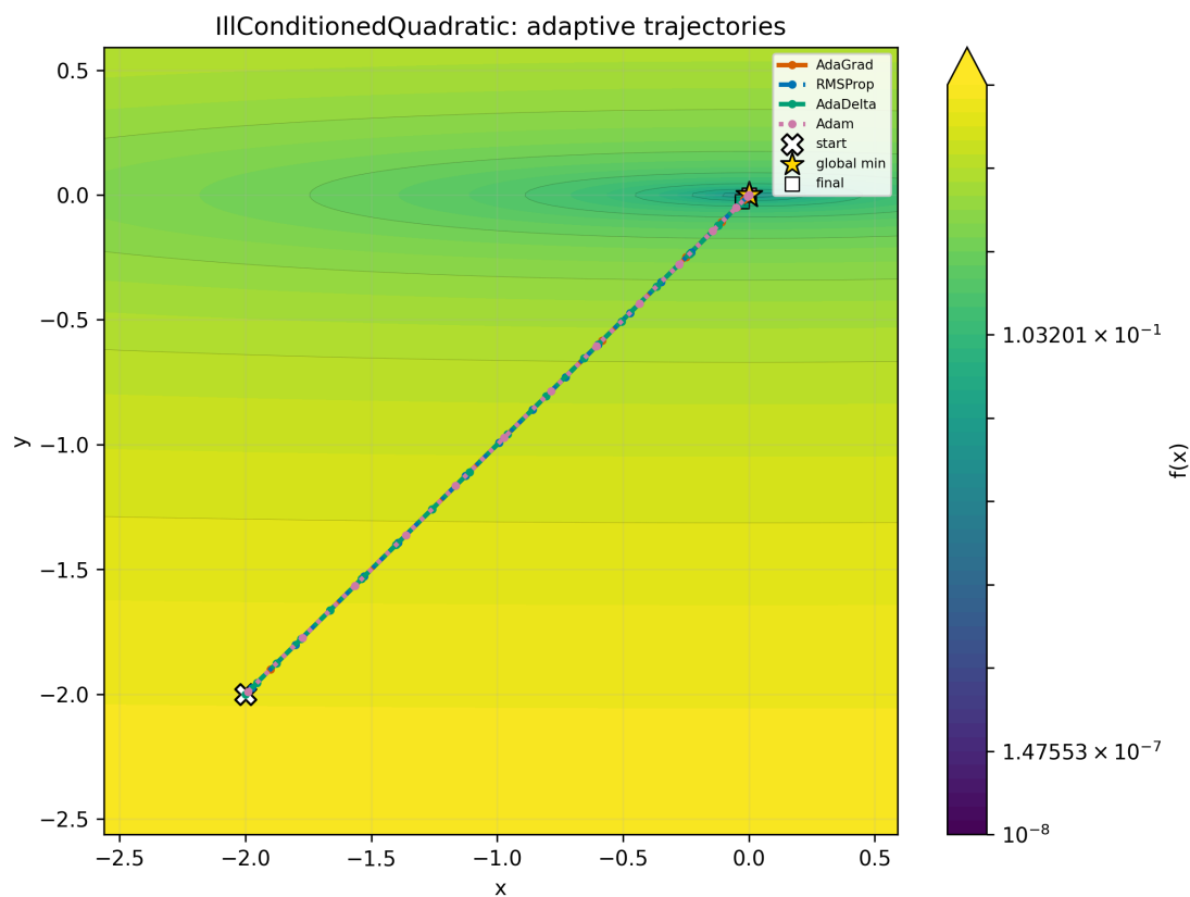
Рис. 22: Адаптивные методы на плохо обусловленной квадратичной функции
