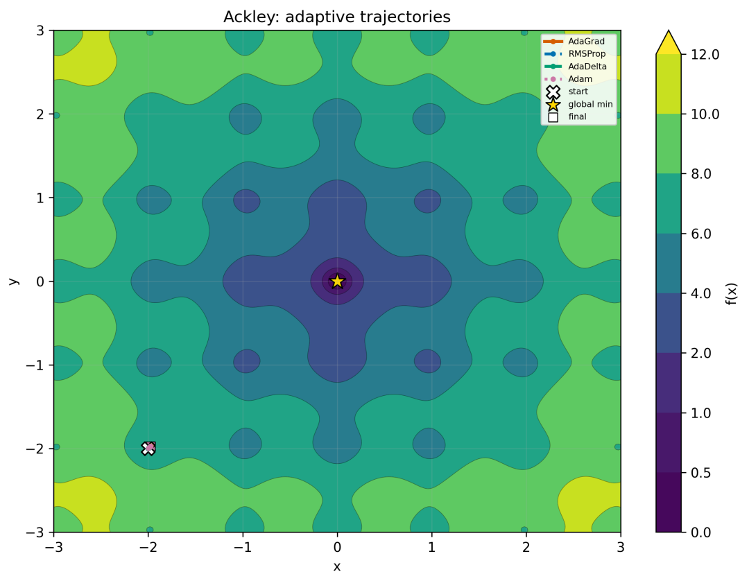
Рис. 34: Ackley, x_0 = (-2.0, -2.0) : адаптивные методы
