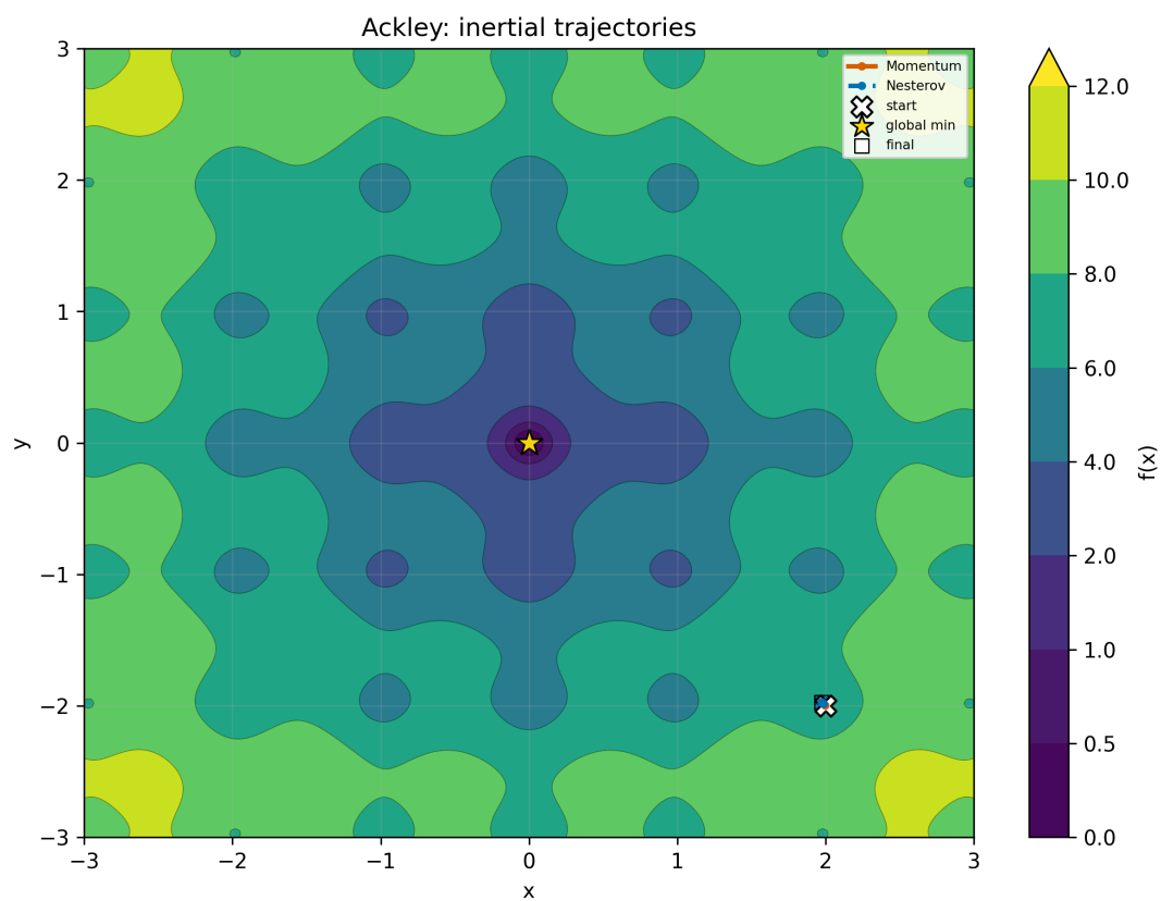
Рис. 35: Ackley, x_0 = (2.0, -2.0) : инерционные методы
