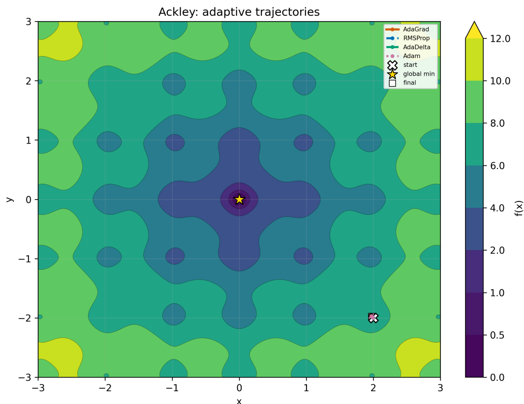
Рис. 36: Ackley, x_0 = (2.0, -2.0) : адаптивные методы
