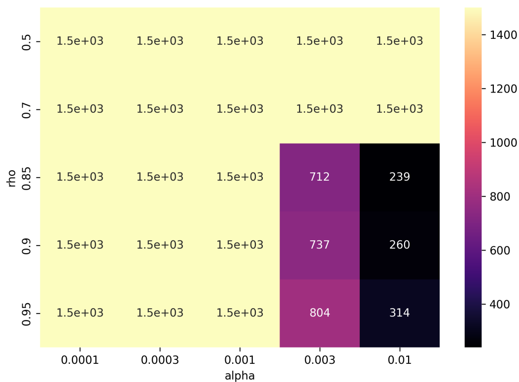
Рис. 13: RMSProp: чувствительность к \alpha и \rho на плохо обусловленной функции
