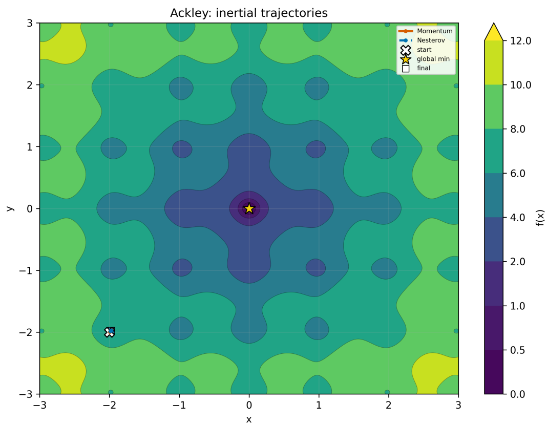
Рис. 33: Ackley, x_0 = (-2.0, -2.0) : инерционные методы
