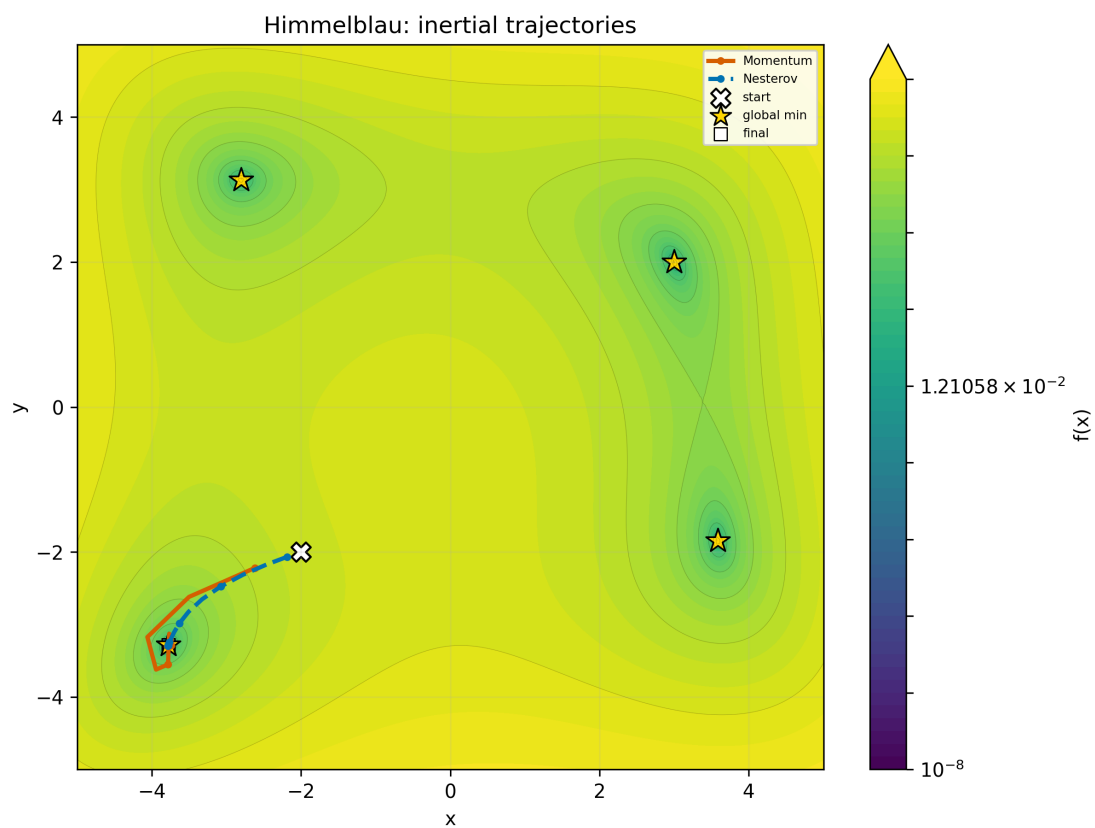
Рис. 39: Himmelblau, x_0 = (-2.0, -2.0) : инерционные методы
