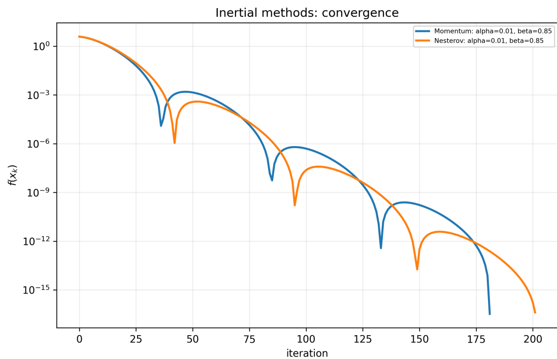
Рис. 19: Инерционные методы: сходимость f(x_k) на хорошо обусловленной функции
