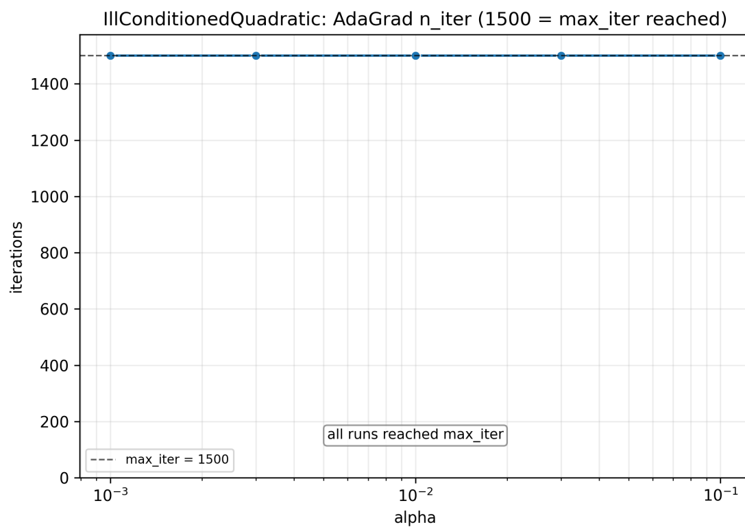
Рис. 11: AdaGrad: чувствительность к \alpha на плохо обусловленной функции
