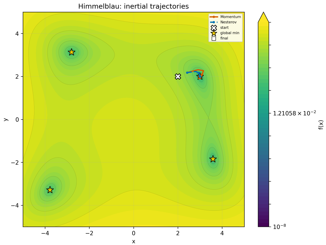
Рис. 37: Himmelblau, x_0 = (2.0, 2.0) : инерционные методы
