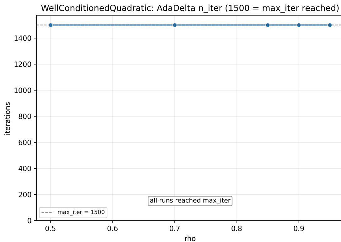
Рис. 6: AdaDelta: чувствительность к \rho на хорошо обусловленной функции
