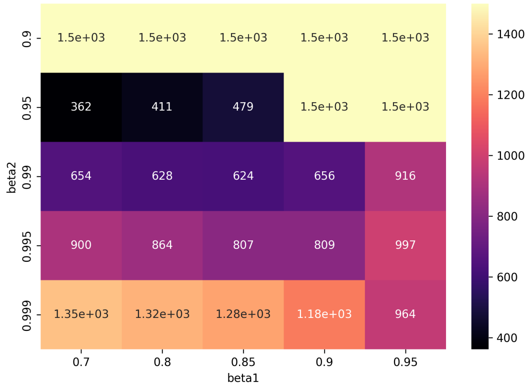
Рис. 16: Adam: чувствительность к \beta_1 и \beta_2 на плохо обусловленной функции
