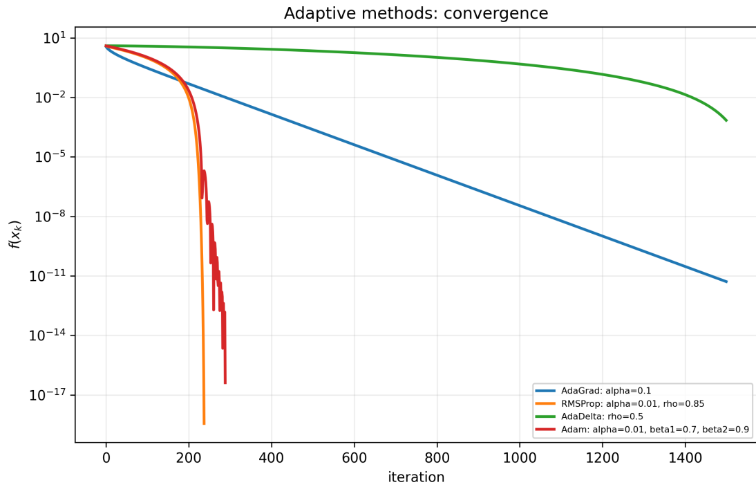
Рис. 20: Адаптивные методы: сходимость f(x_k) на хорошо обусловленной функции
