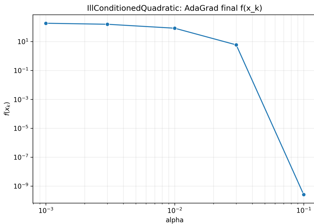
Рис. 12: AdaGrad: конечное значение f(x_k) при разных \alpha на плохо обусловленной функции
