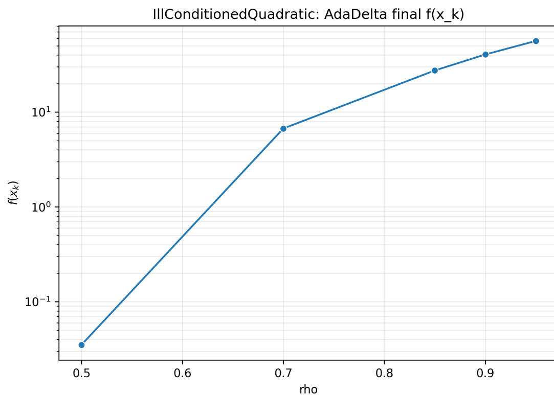
Рис. 15: AdaDelta: конечное значение f(x_k) при разных \rho на плохо обусловленной функции
