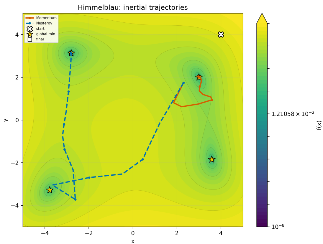
Рис. 41: Himmelblau, x_0 = (4.0, 4.0) : инерционные методы
