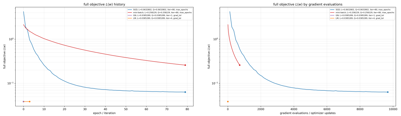
Рис. 7: История полного objective L(w) для near_linear degree 5
