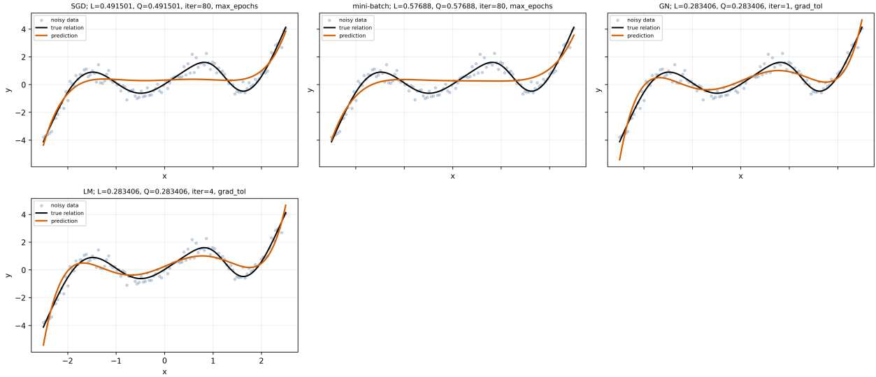
Рис. 6: Аппроксимация nonlinear degree 5 по отдельным методам
