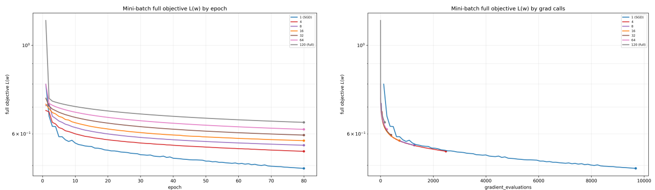
Рис. 11: Влияние размера batch по эпохам и по числу обновлений/градиентных вычислений
