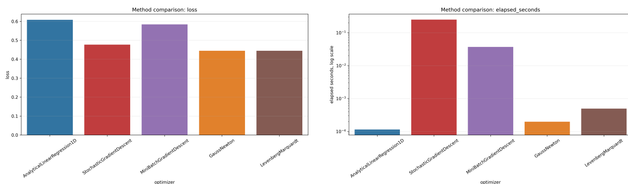
Рис. 21: Сравнение методов по итоговой функции потерь и среднему времени работы
