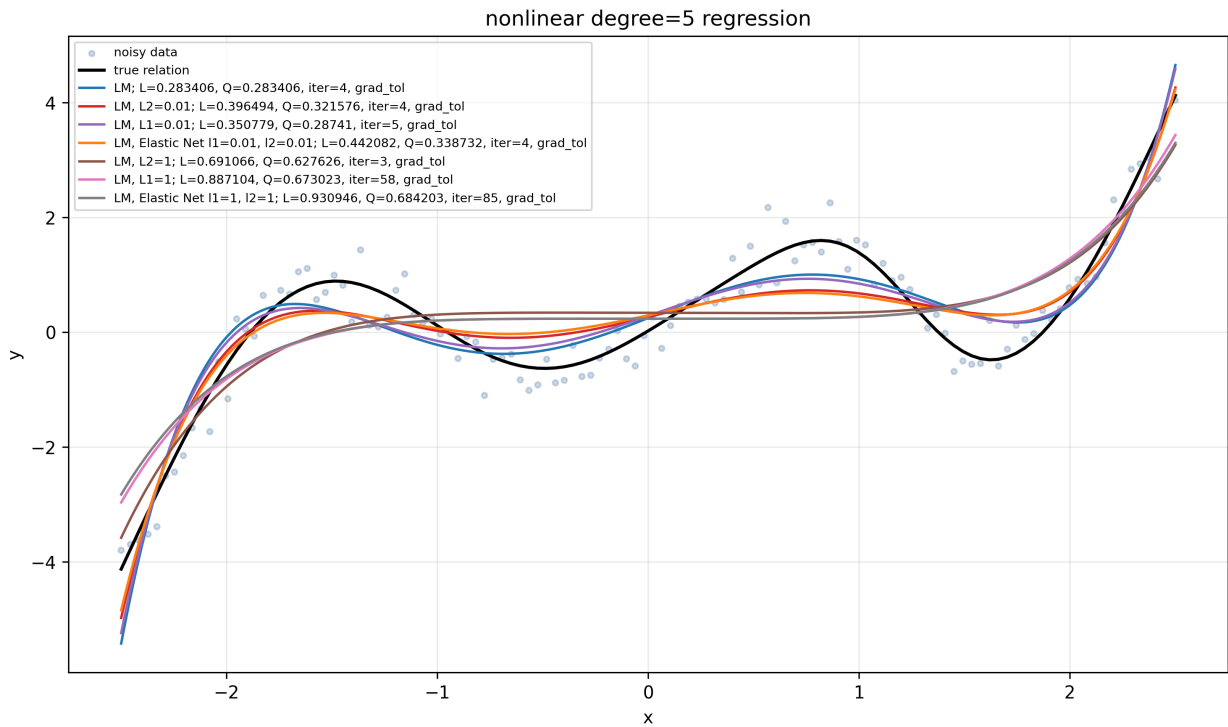
Рис. 18: Аппроксимация nonlinear degree 5 до и после регуляризации
