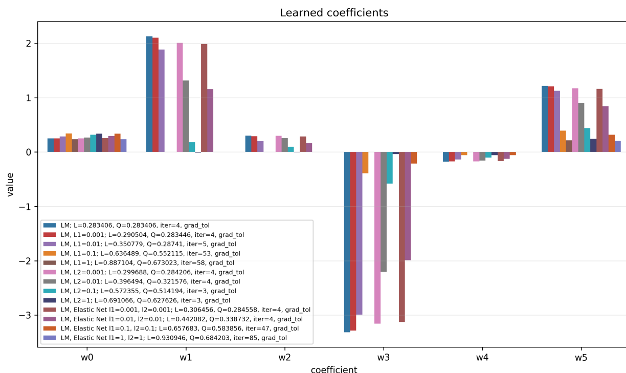
Рис. 20: Коэффициенты при регуляризации
