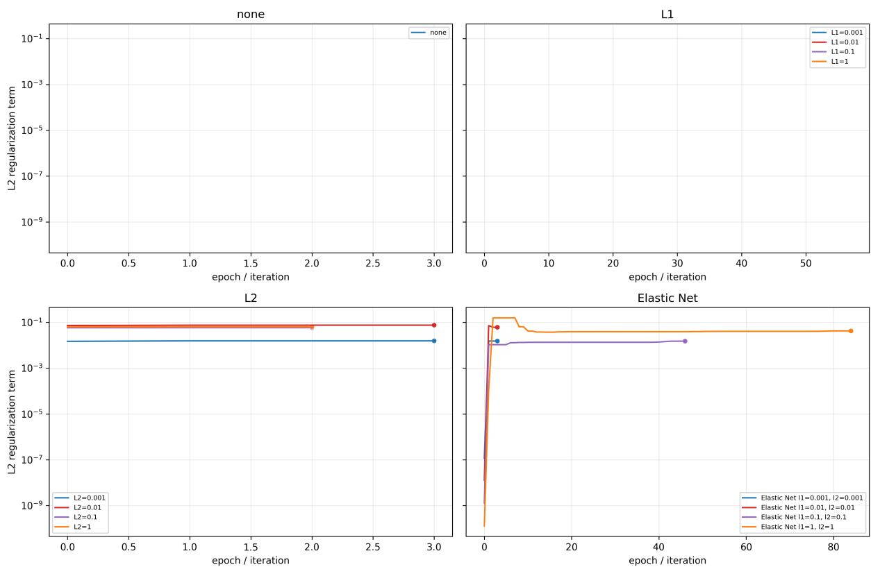
Рис. 17: L2-слагаемое по семействам регуляризации
