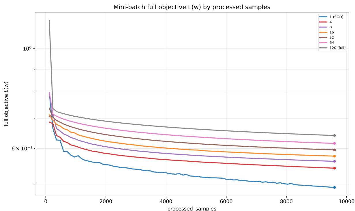
Рис. 12: Влияние размера batch по числу обработанных объектов
