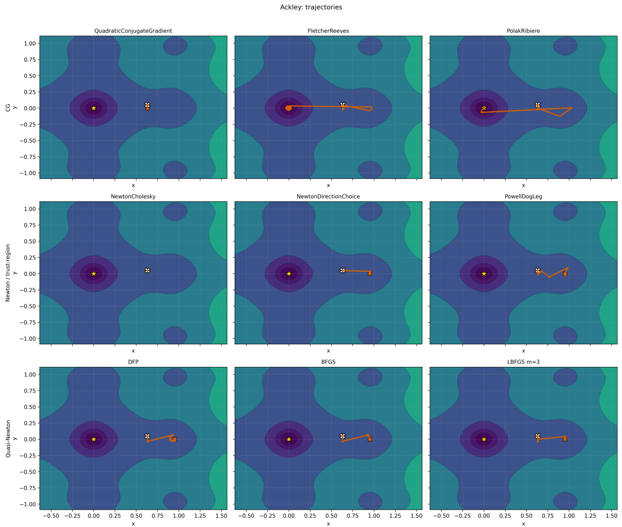
Рис. 4: Траектории на функции Экли из области седловой точки
