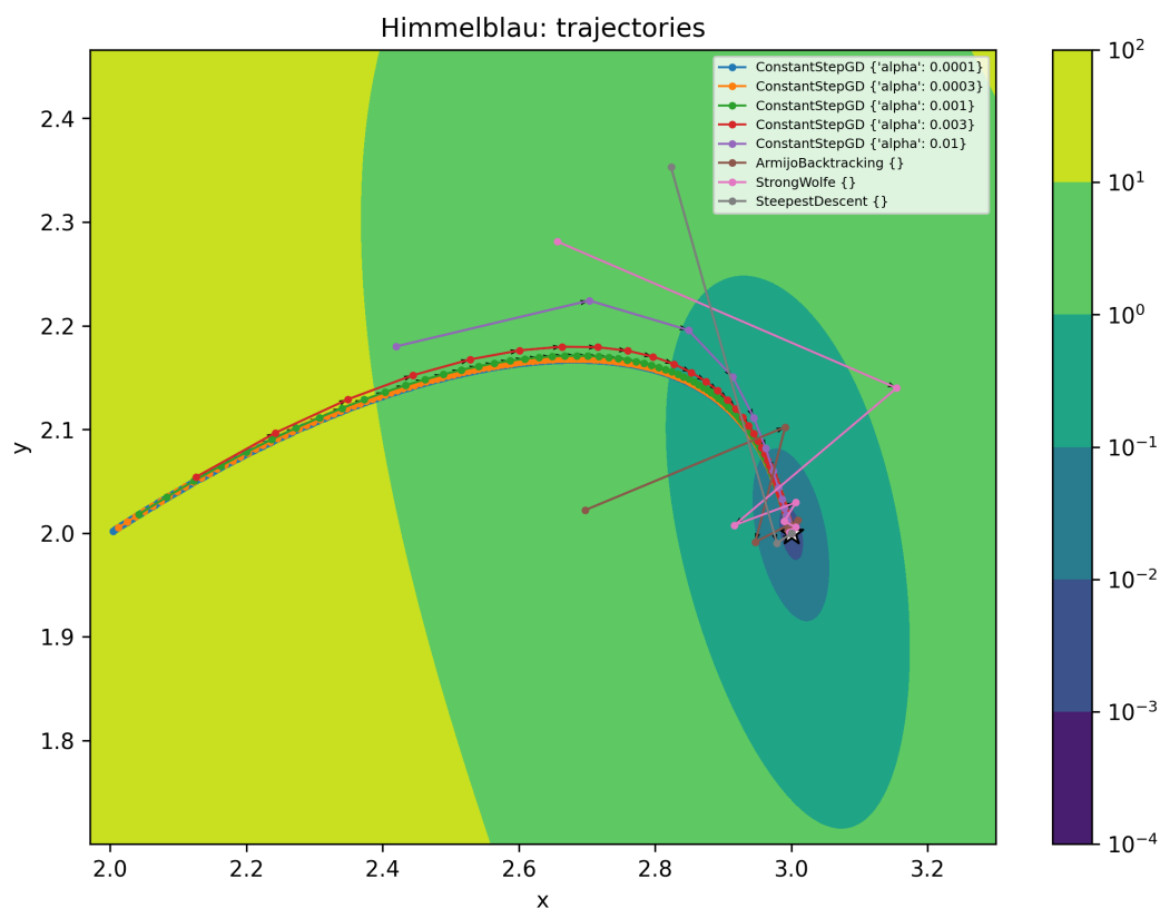
Рис. 9: Траектории методов на функции Химмельблау
