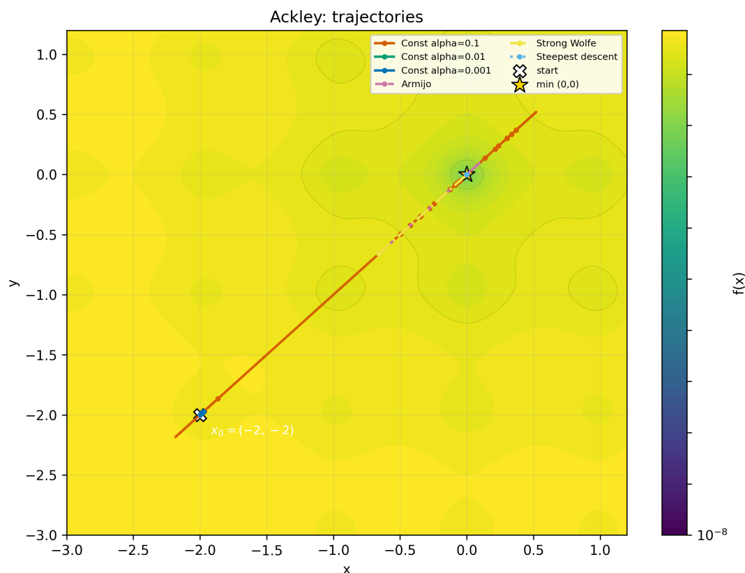
Рис. 8: Траектории методов на функции Экли
