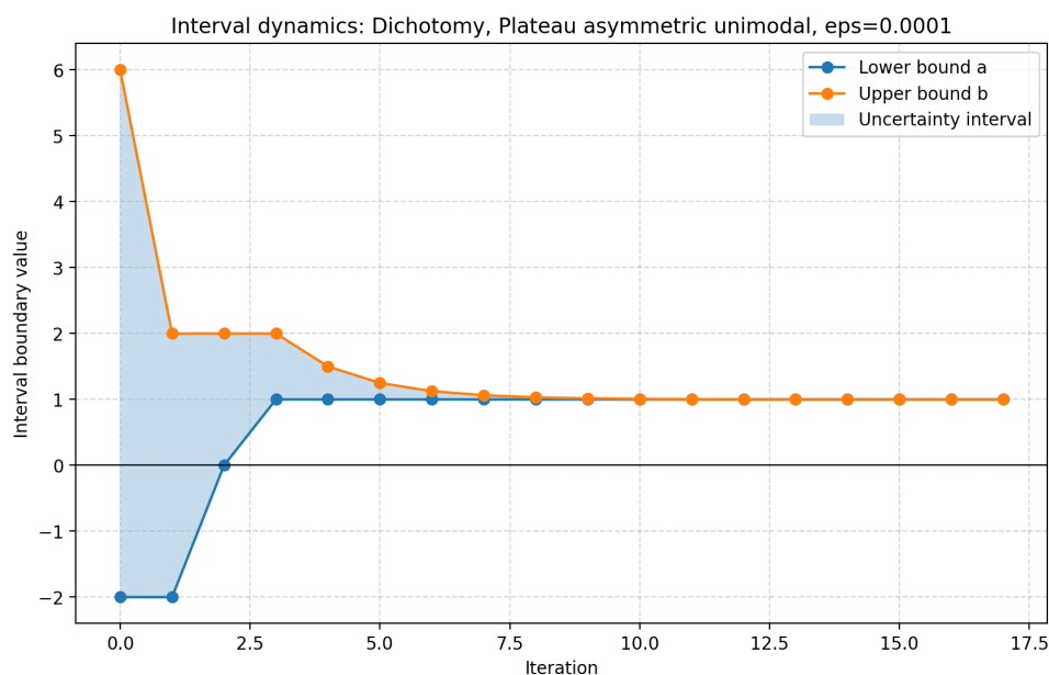
Рис. 5: Динамика интервала неопределенности для метода дихотомии на модифицированной функции с плато и асимметрией
