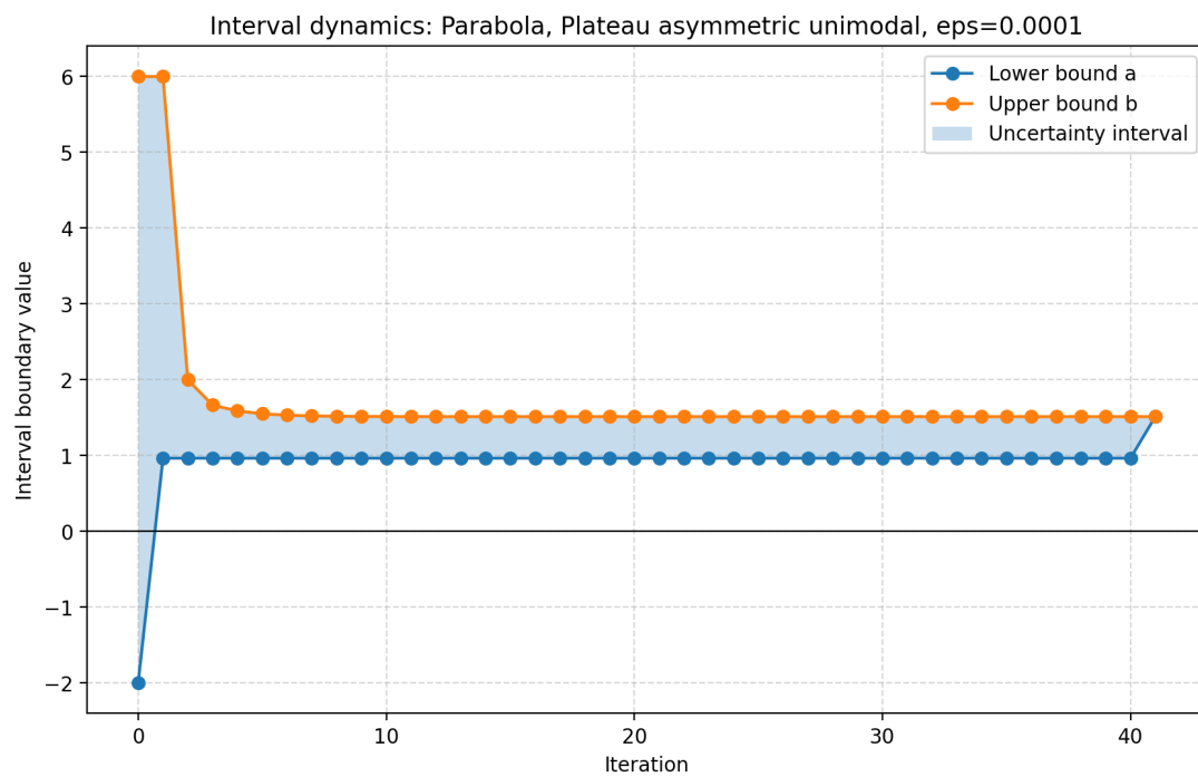
Рис. 14: Динамика интервала неопределенности: метод парабол, функция с плато и асимметрией
