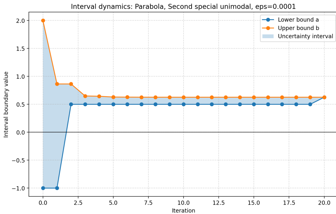
Рис. 20: Динамика интервала неопределенности: метод парабол, асимметричная гладкая функция
