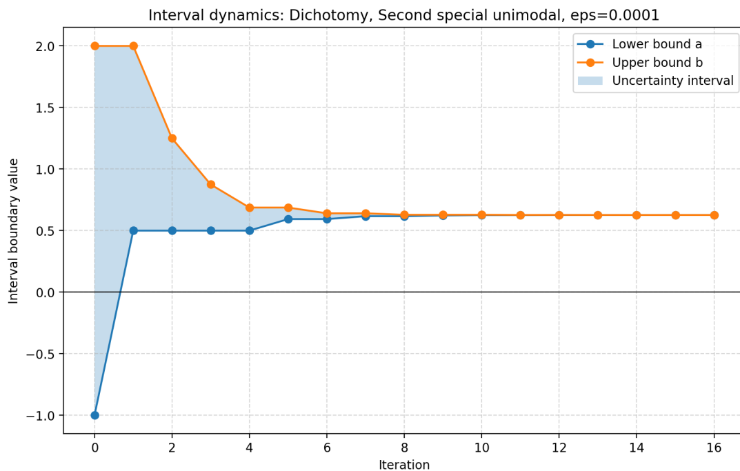
Рис. 17: Динамика интервала неопределенности: метод дихотомии, асимметричная гладкая функция
