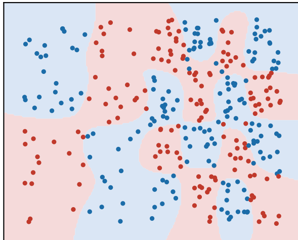
checker_2scale / vb_rbf {'beta': 0.0, 'C': 10.0, 'gamma': np.float64(3.411)}
