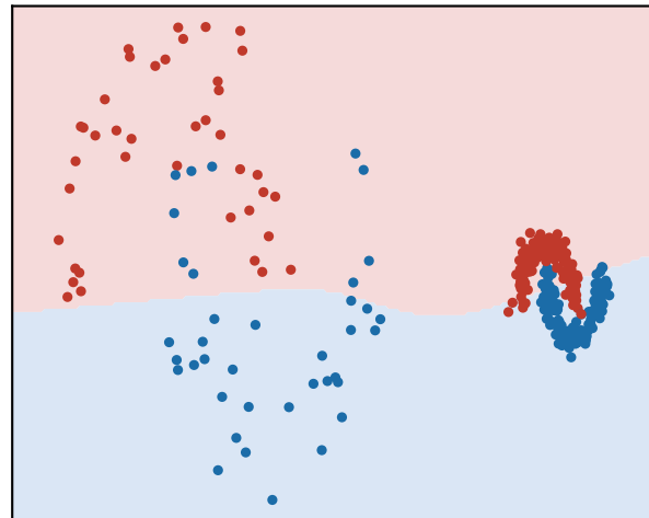
checker_2scale / llsvm {'M': 8, 'C': 10.0}
