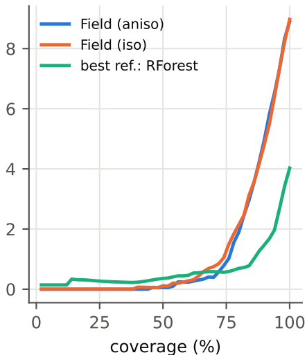
moons-aniso
