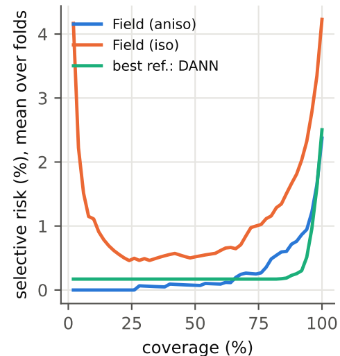
digits
