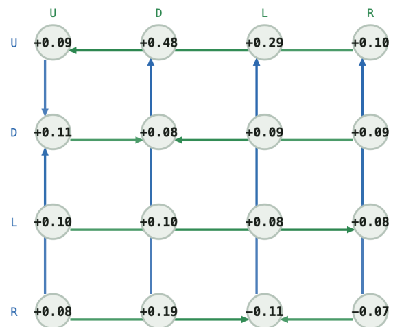
Q matrix -- (0, 1, 1, 1, 0)
