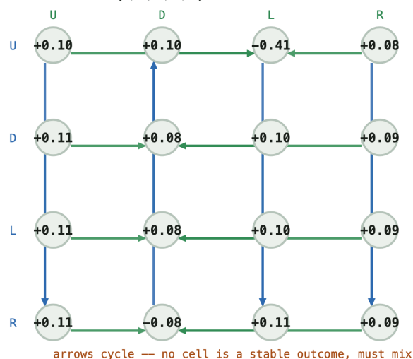
Q matrix -- (0, 0, 1, 1, 0)
