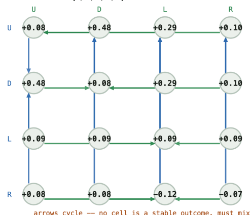
Q matrix -- (0, 2, 1, 2, 0)
