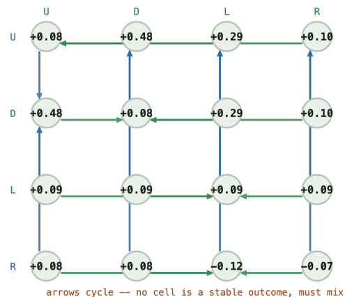
Q matrix -- (0, 2, 1, 2, 0)
